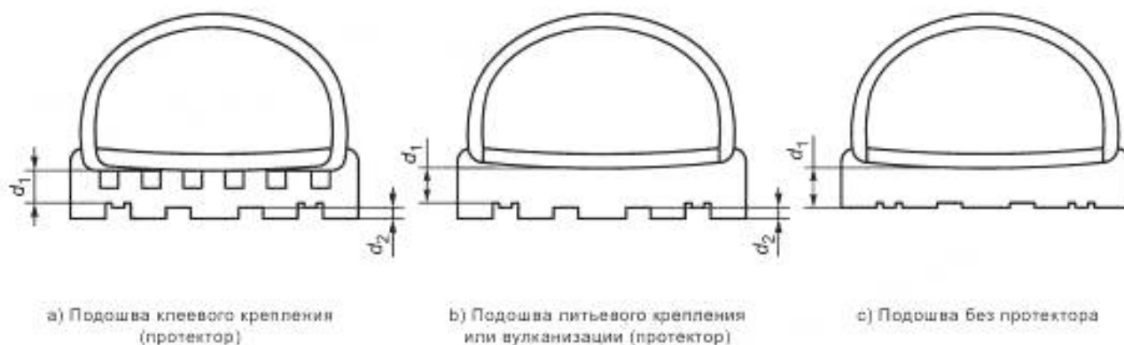
Рисунок 27 — Подошвы клеевого крепления, литьевого крепления, вулканизации
