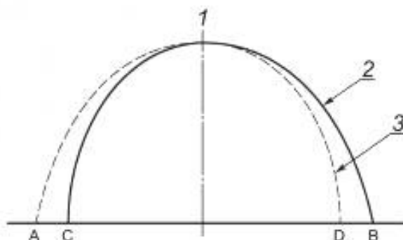
1 — испытательная ось; 2 — правый защитный носок; 3 — левый защитный носок
