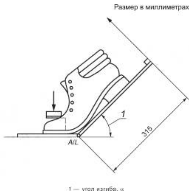
Рисунок 32 — Угол изгиба
