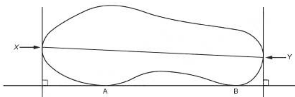
Рисунок 5 — Испытательная ось обуви
