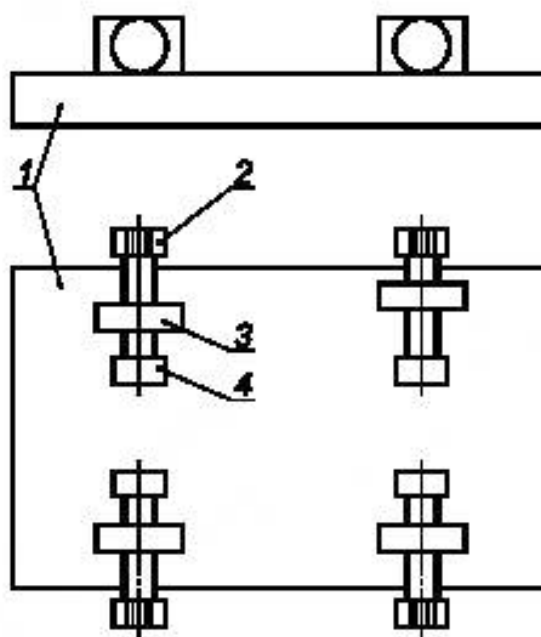
1 — опорная плита; 2 — винт; 3 — винтовой зажим; 4 — прижимная пластина
