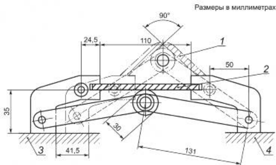
1 — испытуемая проба в максимально изогнутом положении; 2 — испытуемая проба до изгиба; 3 — подвижная опора; 4 — неподвижная опора
