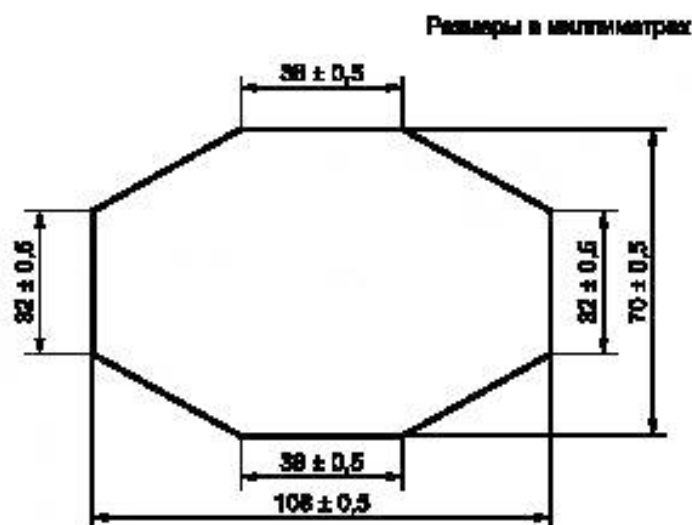
Рисунок 23 — Испытуемая проба для испытания на изгиб
