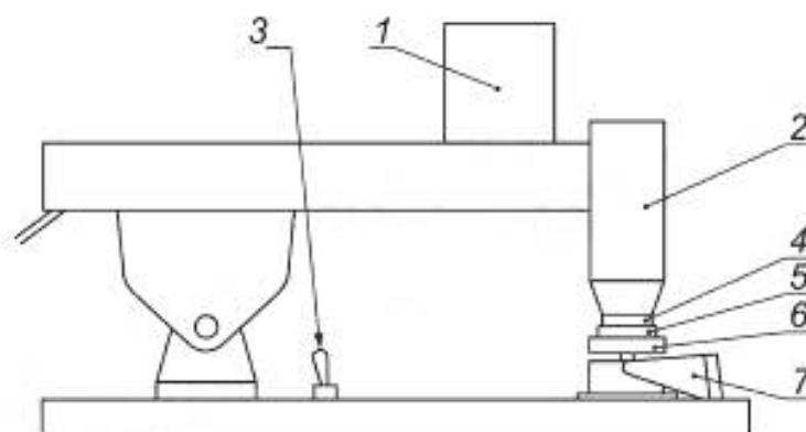
1 — груз; 2 — установленные в корпус нагревательные блоки, включающие устройство измерения температуры; 3 — вкл/выкл тумблер; 4 — квадратный конец медного бита; 5 — испытуемую пробу; 6 — самовыравнивающаяся платформа для испытуемого образца; 7 — шарнирная теплоизолированная опора
