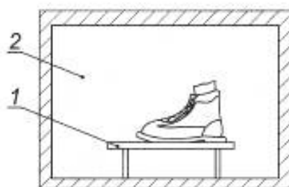
1 — медная пластина (см. 5.13.1.5); 2 — термоконтейнер
