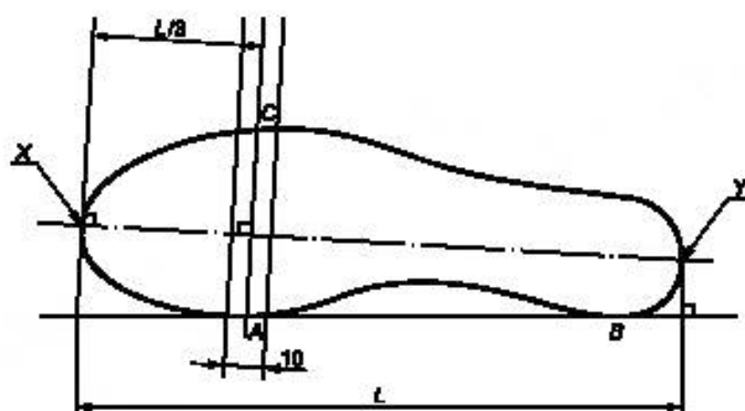
Рисунок 30 — Положение линии изгиба на подошве
