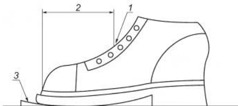
1 — точка удара; 2 — расстояние из таблицы 9; 3 — клин
