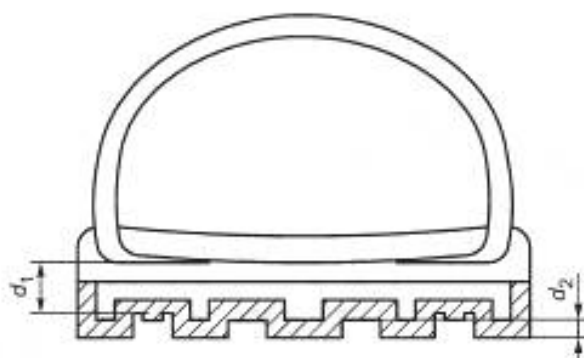
Рисунок 28 — Многослойная подошва (протектор)
