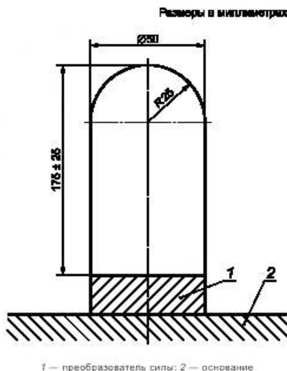
Рисунок 21 — Наковальня и основание
