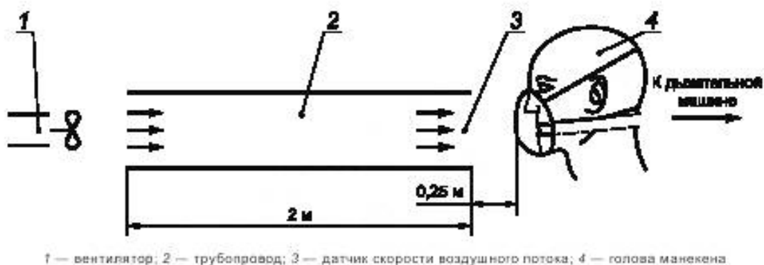
Рисунок 10 — Схема испытания и подачи воздуха для определения содержания диоксида углерода
