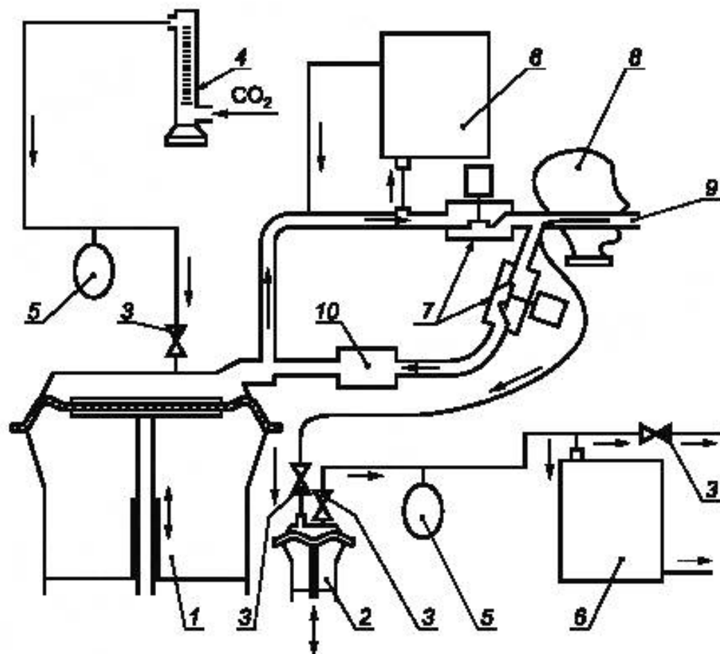
1 — дыхательная машина; 2 — вспомогательное клетчатое; 3 — обратный клапан; 4 — расходомер; 5 — компенсатор; 6 — анализатор диоксида углерода; 7 — сопловидные клапаны; 8 — голова манекена; 9 — трубка для отбора проб из вдыхаемого воздуха; 10 — поглотитель диоксида углерода
