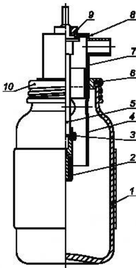
1 — стеклянный сосуд с навинчивающейся крышкой; 2 — горло; 3 — волокнистая прокладка (наружный диаметр — 4,5 мм, внутренний диаметр — 2 мм, толщина прокладки — 0,8 мм); 4 — втулка; 5 — стержень; 6 — резиновая прокладка; 7 — головка втулки; 8 — резиновая прокладка (наружный диаметр — 25 мм, внутренний диаметр — 10 мм, толщина — 1,5 мм, уплотнитель для герметизации); 9 — гайка; 10 — навинчивающаяся крышка
