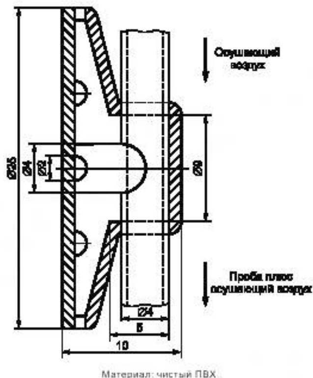
Рисунок 5 — Пробоотборник
