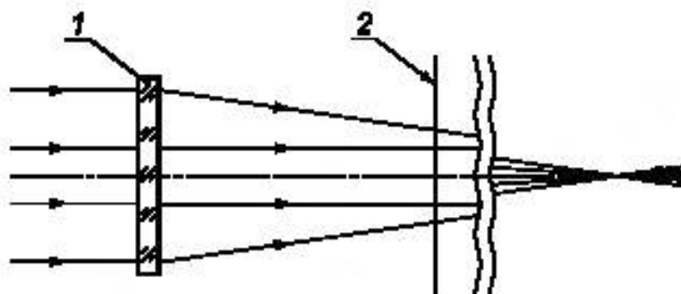
1 — испытуемый смотровой элемент; 2 — плоскость измерений
