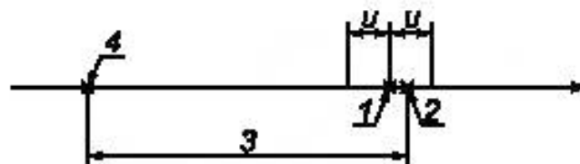
1 — результат измерения; 2 — верхнее предельное значение параметра; 3 — интервал допустимых значений параметра; 4 — нижнее предельное значение параметра
