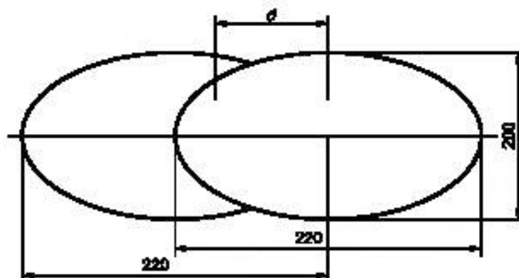
Рисунок 5 — Контрольные эллипсы для определения поля зрения
