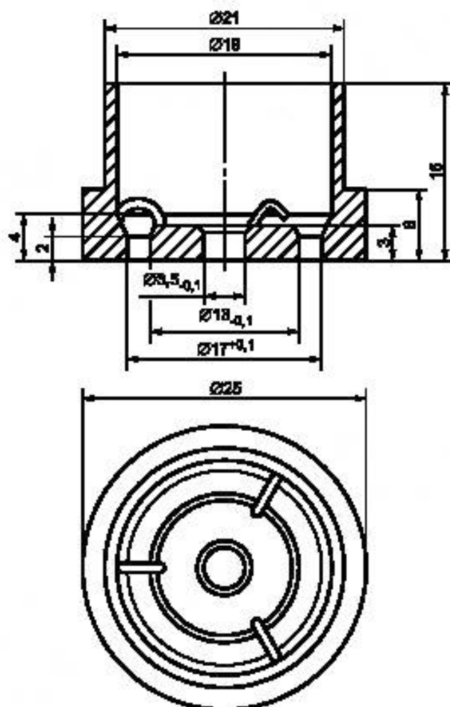
Рисунок 18 — Выходное сопло контейнера
