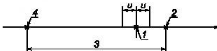
1 — результат измерения; 2 — верхнее предельное значение параметра; 3 — интервал допустимых значений параметра; 4 — нижний предел значений параметра
