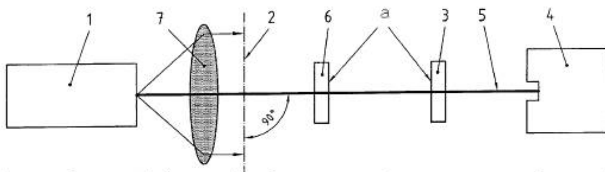
1 – лазер; 2 – опорная (референтная) ось; 3 – поляризатор; 4 – приемник излучения; 5 – лазерный пучок; 6 – четвертьволновая пластина; 7 – коллиматор; а – вращение в пределах 180°
