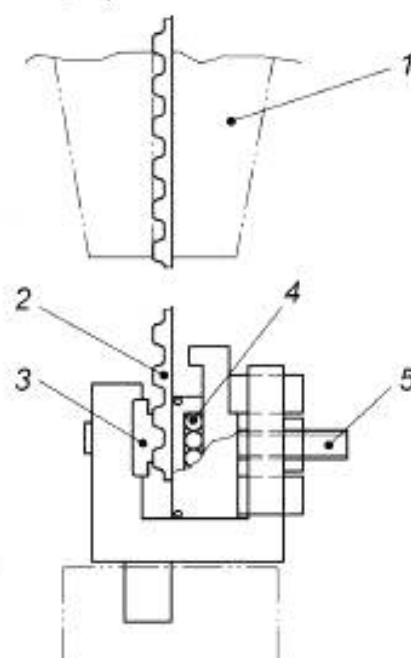
Рисунок 4 — Устройство для определения прочности зубьев на сдвиг
