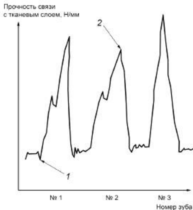
1 — основание зуба; 2 — пик разрыва в теле зуба
