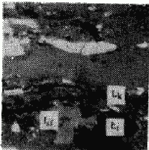
Отраженный свет Масляная иммерсия 600 \times L sl — семифлюзит L k — кутинит L r — резинит Черт. 13
