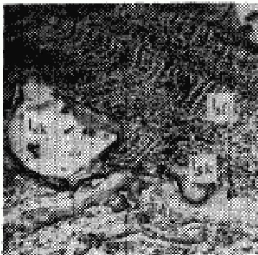
Отраженный свет 100 \times I 10f — семифюзинит I 10sk — склеротинит Черт. 7
