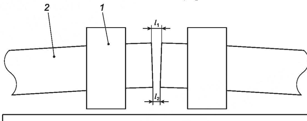
а) Имеются опорные ролики |l_1 - l_2| \leq 0,5 мм
