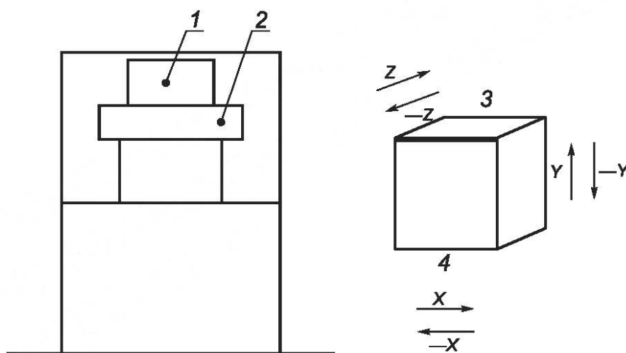
Рисунок С.1 — Испытания на ударпрочность
