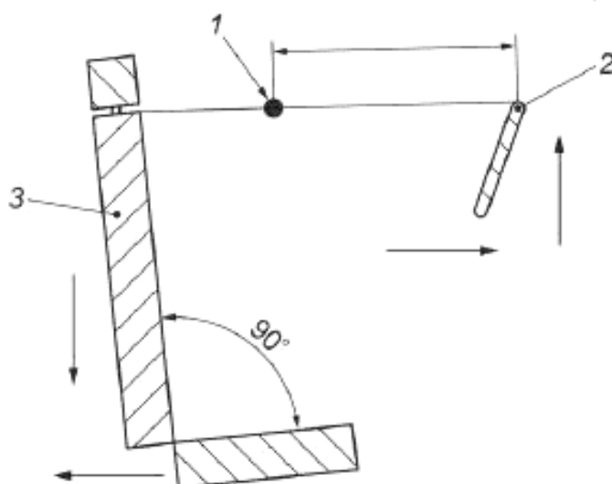
1 – точка отбора проб; 2 – руль; 3 – кресло с подголовником
