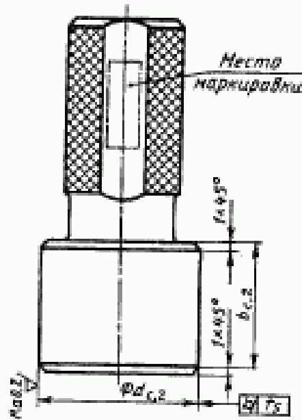
Рисунок 5 — Калибр-пробка сплошная для d'_{c,2} \leq 80 мм
