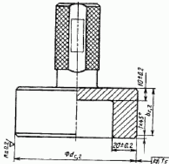
Рисунок 6 — Калибр-пробка с глухим отверстием для d'_{c,2} > 80 мм
