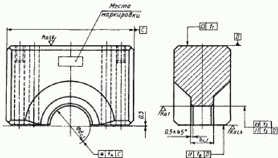
Рисунок 3 — Верхний полувкладыш контрольного блока
