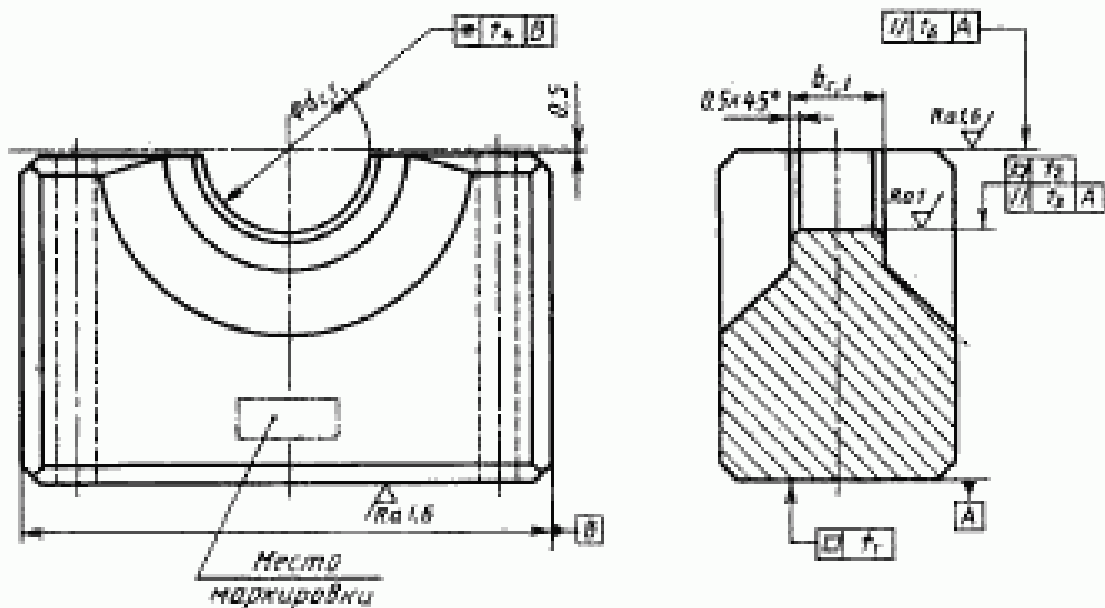
Рисунок 4 — Нижний полувкладыш контрольного блока
