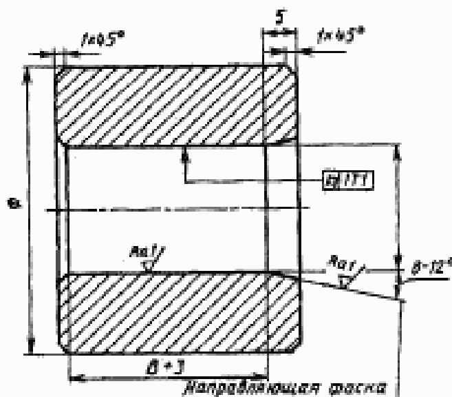
Рисунок 7 — Кольцевой калибр
