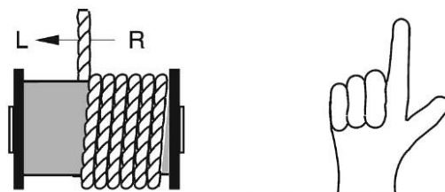
Рисунок В.1а — Канат правой свивки — подмотка
