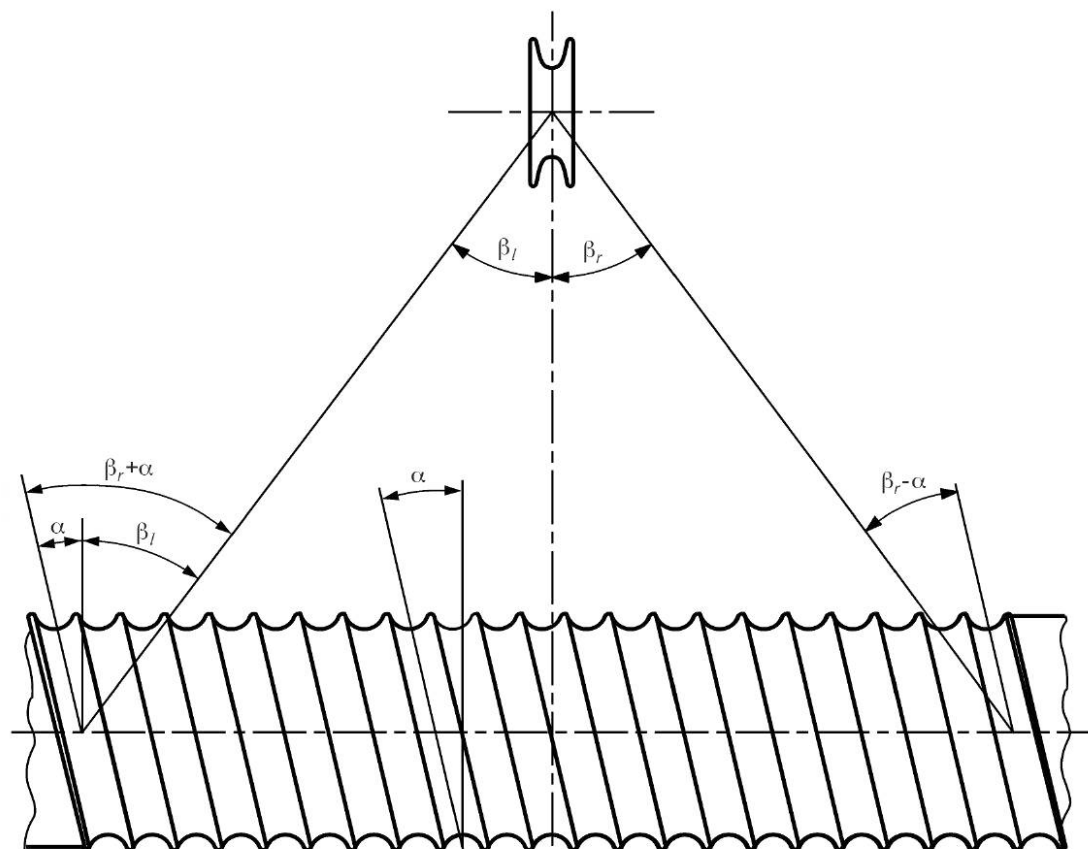
Рисунок В.2 — Угол наклона каната и угол наклона желоба
