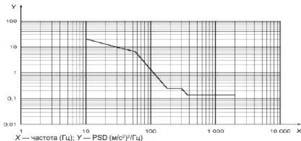
Рисунок 12 — Распределение PSD по частоте колебаний
