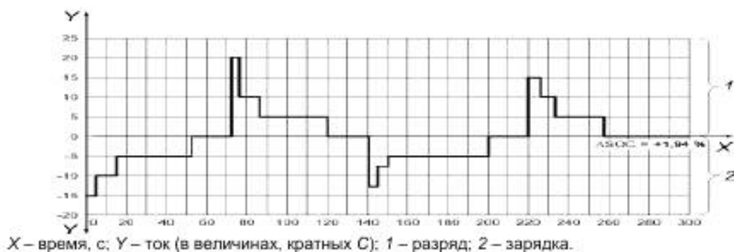
Рисунок 8 — Режим по току для циклического испытания на долговечность. Режим постепенной зарядки.
