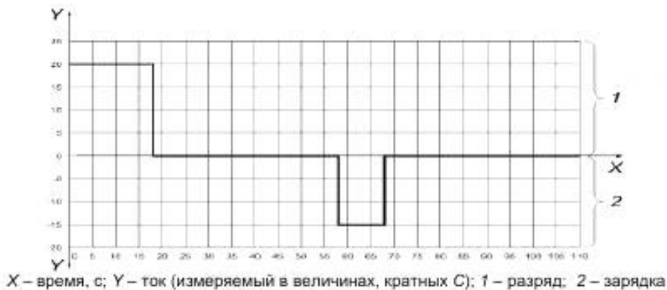
Рисунок 5 — Снятие характеристик мощности в импульсе (график по току)
