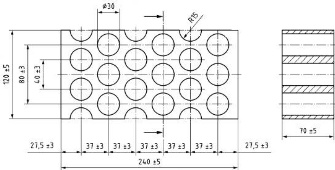
Рисунок В.1 — Экран для испытания на огнестойкость
