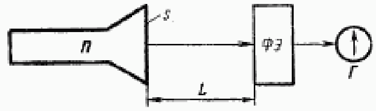
П — электронно-лучевой прибор; S — площадь раstra; L — расстояние между расстром и светочувствительной поверхностью фотоэлемента; ФЭ — селеновый фотоэлемент, спектральная чувствительность которого должна соответствовать ГОСТ 11093—64; Г — гальванометр.
