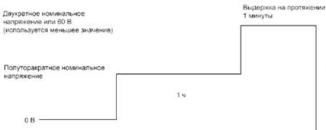
Рисунок 2 — Цикл испытания на воздействие повышенных электрических напряжений
