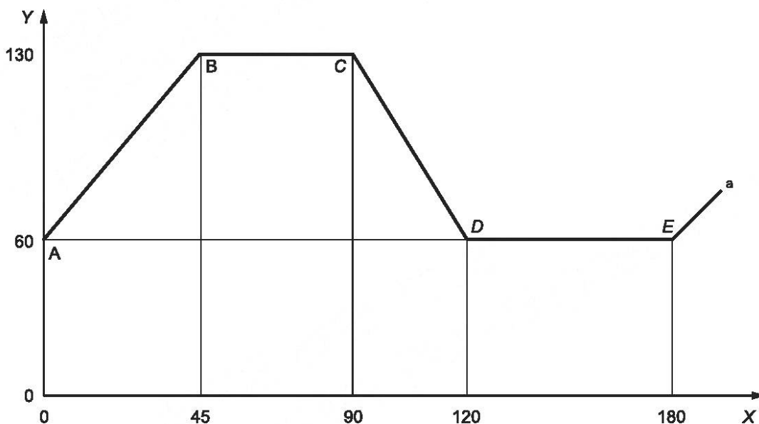
Рисунок 1 — Термоциклы
