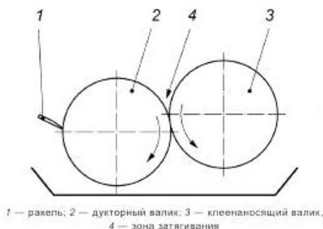
Рисунок 28 — Валковый клеевой аппарат с ракелем на дукторном валке
