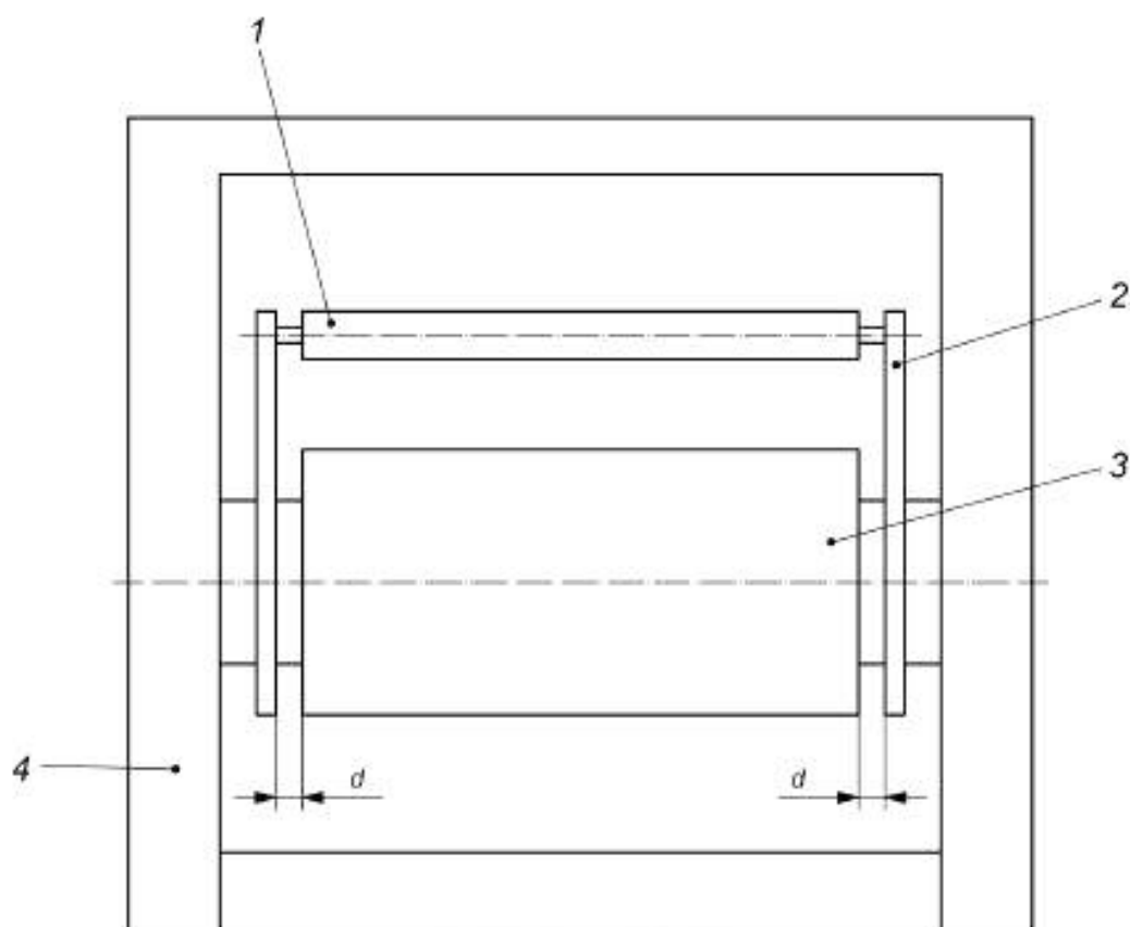
1 — обхватывающий вал; 2 — поворотный рычаг; 3 — нагревательный цилиндр; 4 — станка машины; d — расстояние между нагревательным цилиндром и поворотным рычагом
