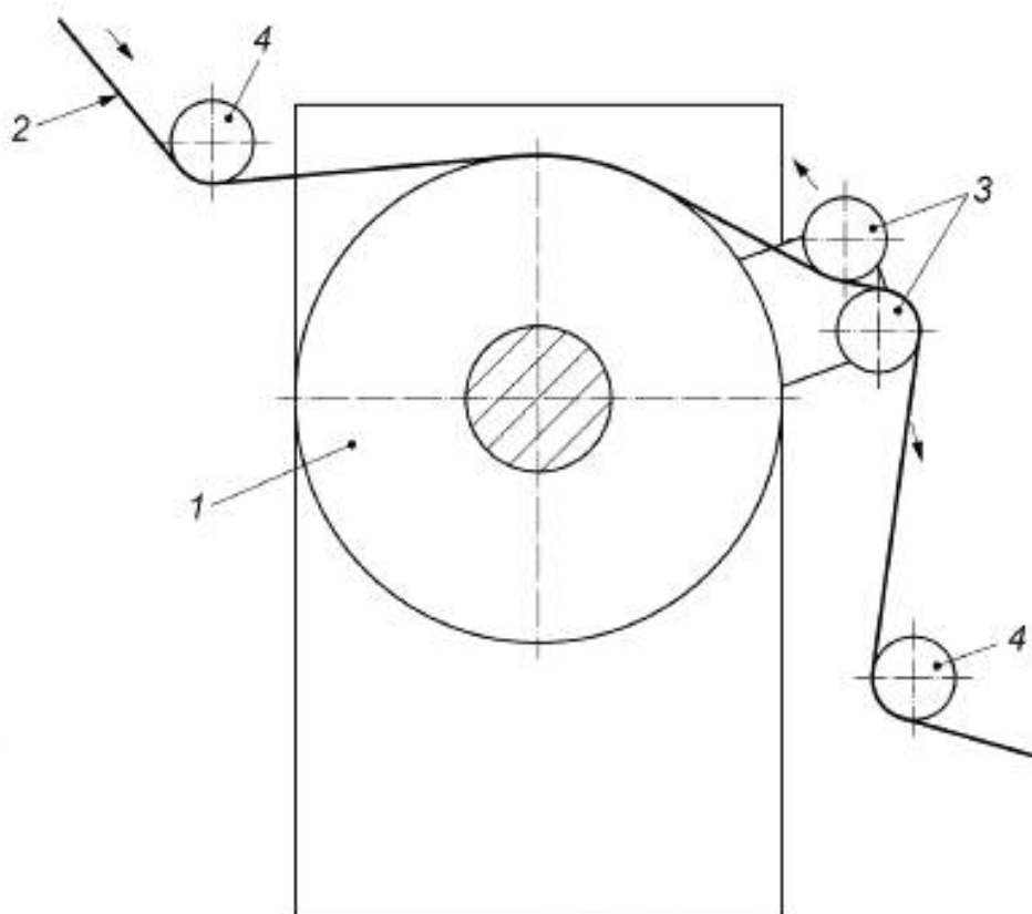
1 — нагревательный цилиндр; 2 — бумажное полотно; 3 — обхватывающие валики; 4 — направляющие валики
