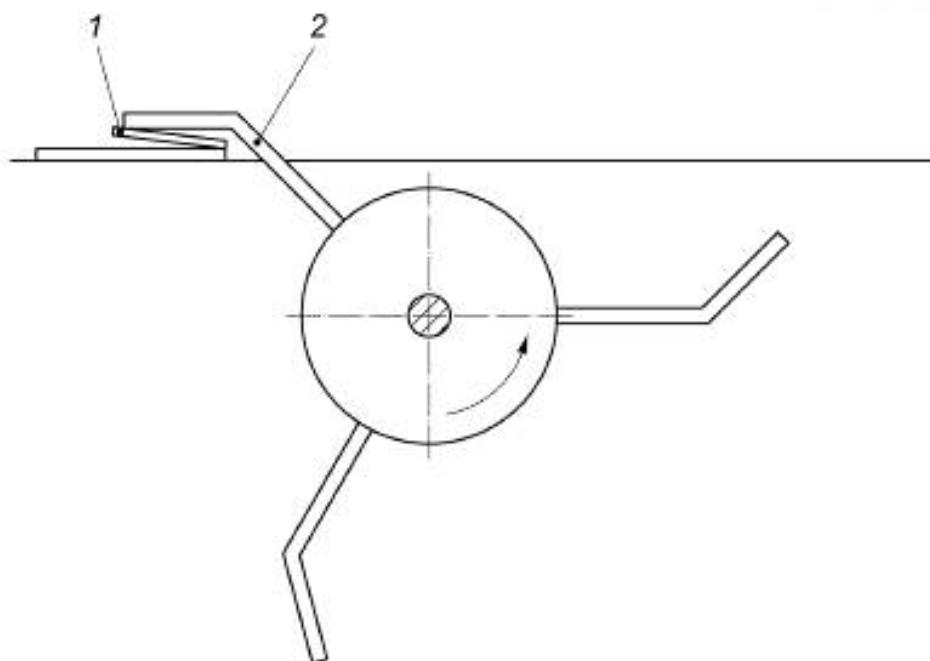
1 — сфальцованная заготовка; 2 — фальцевальный крюк
