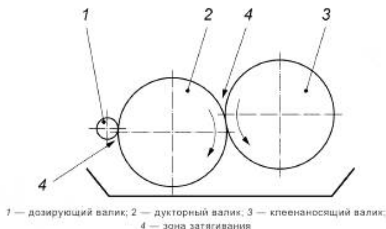
Рисунок 27 — Валковый клеевой аппарат с дозирующим валком
