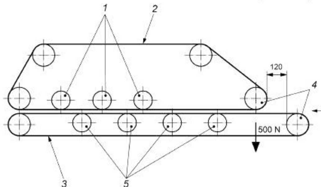
Рисунок 20 — Секция обжимки
