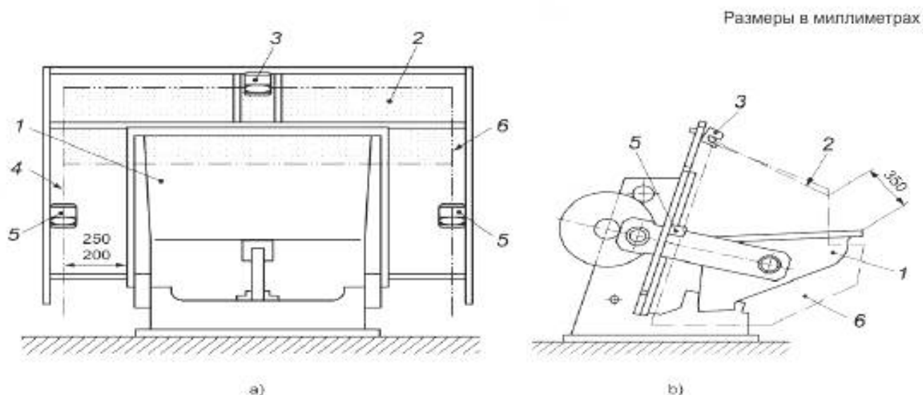
1 — подвижный титель; 2 — сканируемая зона наверху; 3 — лазерный сканер для сканируемых зон наверху; 4 — неподвижное защитное ограждение; 5 — лазерный сканер для сканируемых боковых зон; 6 — боковые зоны сканирования
