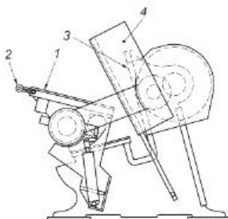
1 — подвижный тигель; 2 — нажимное СПУ подвижного тигля; 3 — плоскость высежки; 4 — предохранительное устройство
