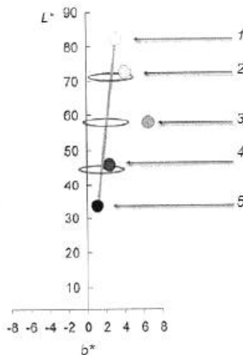
1 — бумага; 2 — серый в светах, в данном случае в пределах допусков; 3 — серый в полутонах, в данном случае вне допусков; 4 — тени, в данном случае в пределах допусков; 5 — G_{max} , полученное при максимальной сумме значений тона
