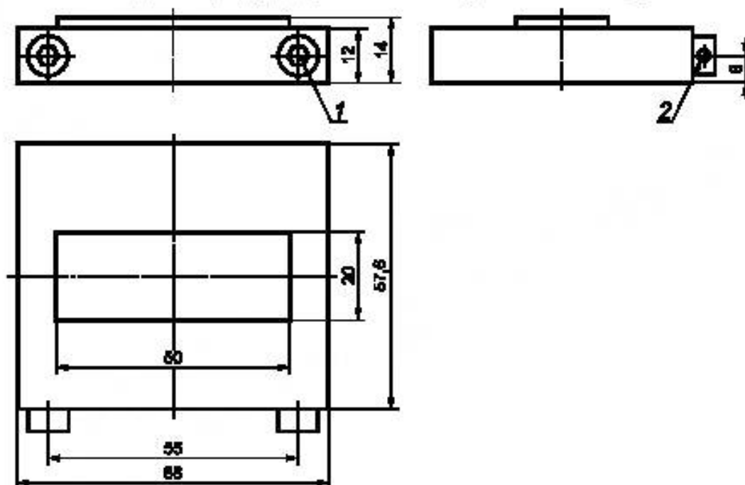
Рисунок В.1 — Плита
