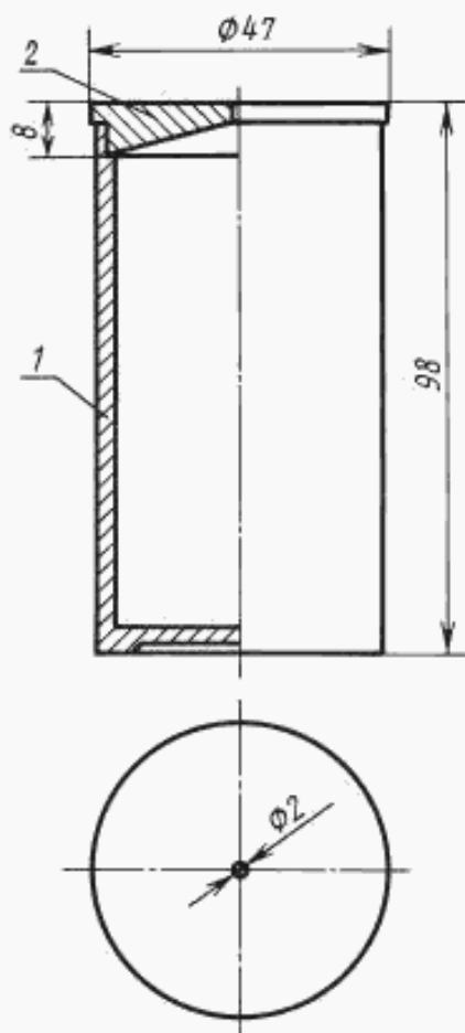
1 — корпус; 2 — крышка
