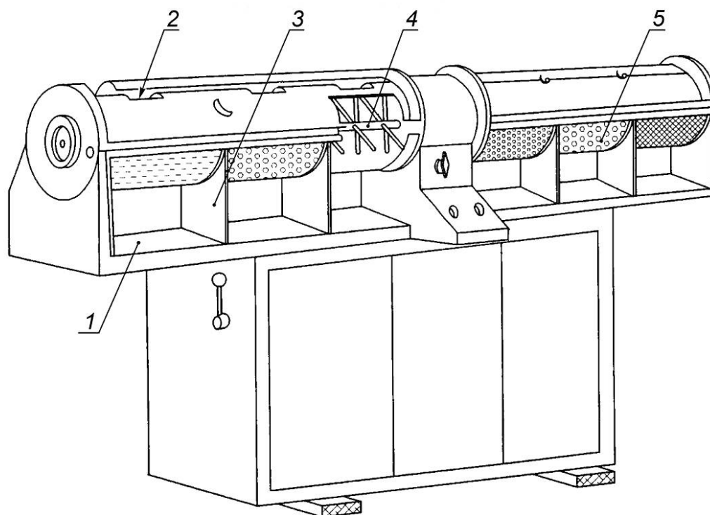
1 — рабочая камера; 2 — загрузочная воронка; 3 — перегородка; 4 — вал с колодками; 5 — сито
