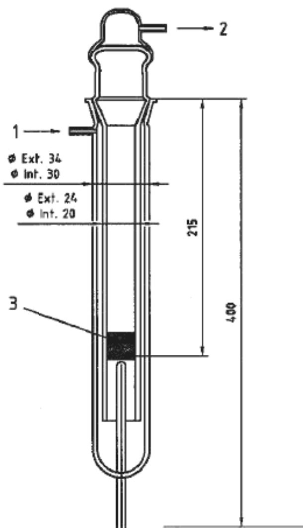
Рисунок 3 – Трубчатый реактор с анализируемой пробой
