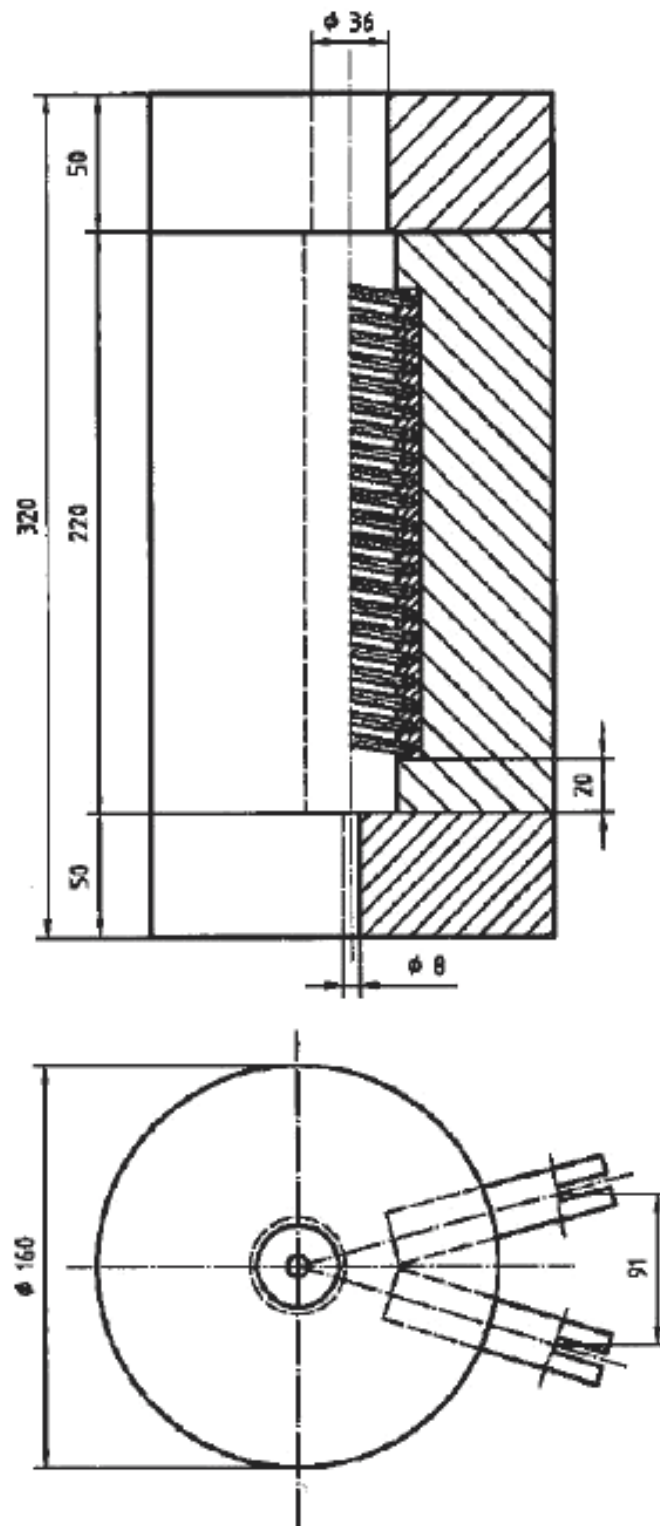
Рисунок 2 — Характеристики и размеры типовой печи
