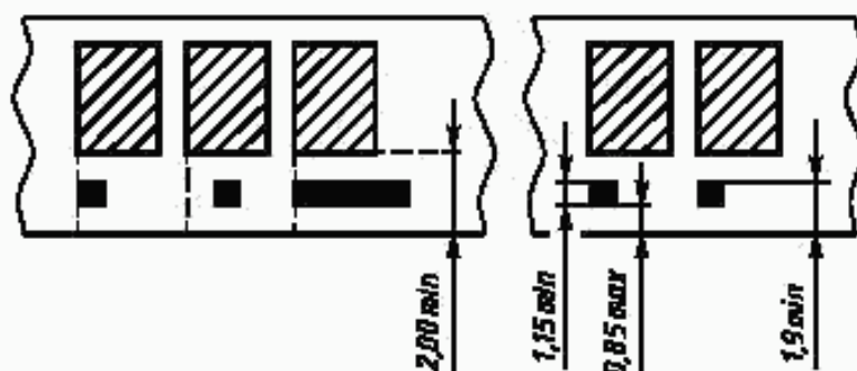
Рисунок 1 — Размещение счетной метки в зоне кодирования
