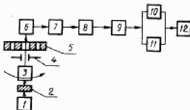
Блок-схема установки
