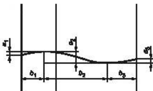
Рисунок 8 — Местный диагональный перекося (модель по трем треугольникам)
