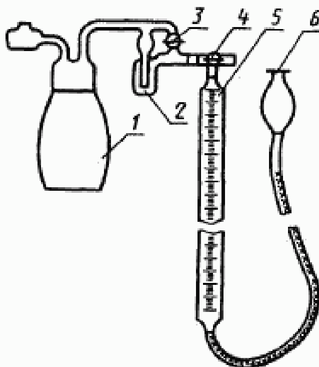
Прибор для определения массовой доли воды
