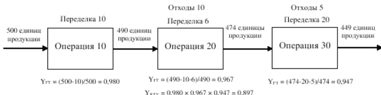
Рисунок 3 – Пример вычисления вероятности штучного сквозного выхода
