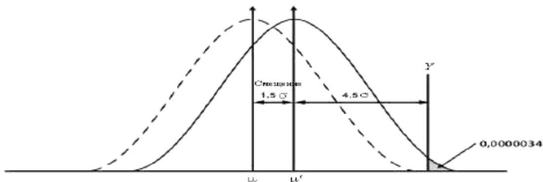
Рисунок 2 – Получение числа сигм
