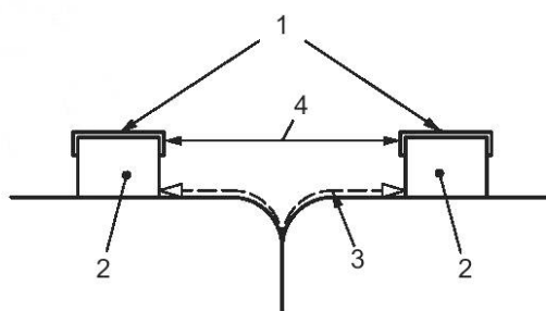
Рисунок 2 — Путь утечки и воздушный зазор
