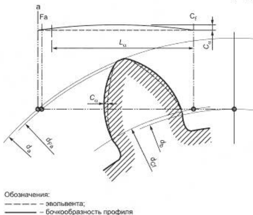
Рисунок В.1 — Бочкообразность профиля
