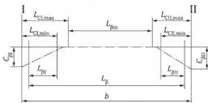
I — базовый торец; II — не базовый торец; C_{II} — значение от среза торца; C_{III} — значение от среза торца; L_{CI,max} — максимальная длина от среза торца; L_{CI,min} — минимальная длина от среза торца; L_{CII,max} — максимальная длина от среза торца; L_{CII,min} — минимальная длина от среза торца; L_{\beta I} — зона среза торца; L_{\beta m} — средняя зона направления линии зуба; L_{\beta II} — зона среза торца
