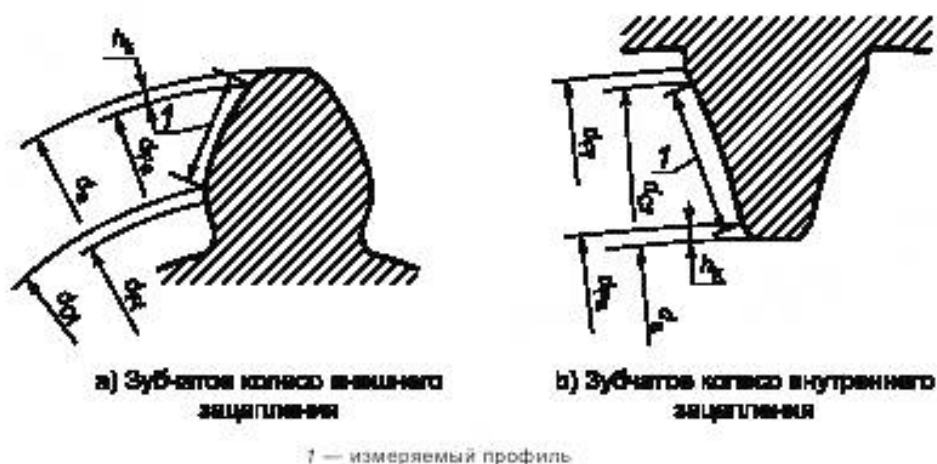
Рисунок 3 — Измеряемый профиль
