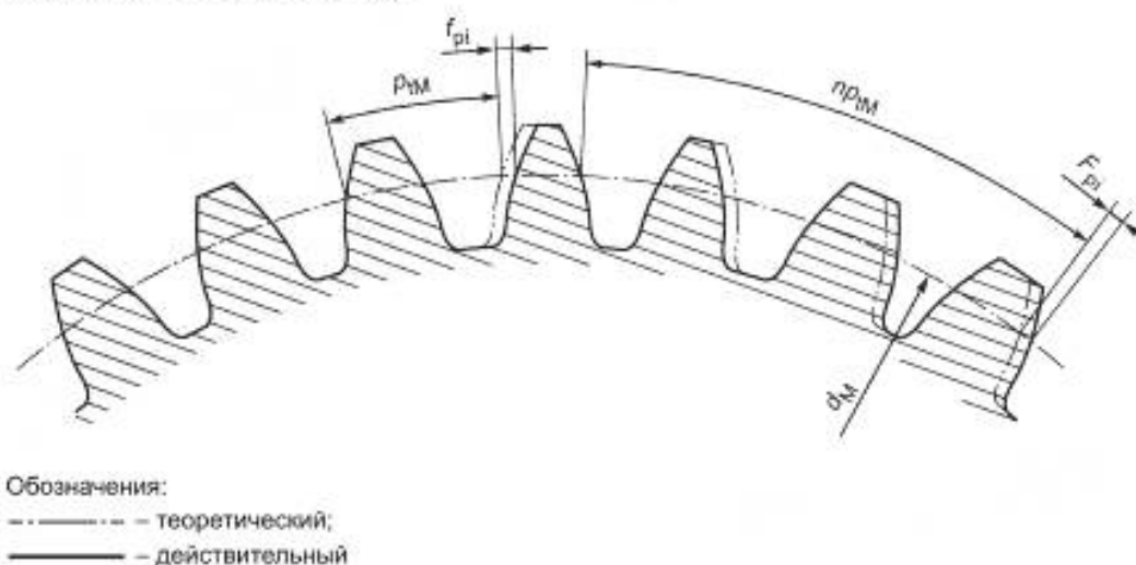
Рисунок 2 — Погрешности шага
