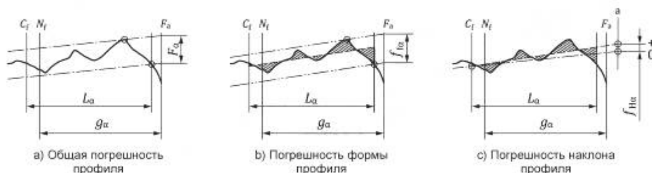
Рисунок 4 — Погрешности профиля с немодифицированной эвольвентой
