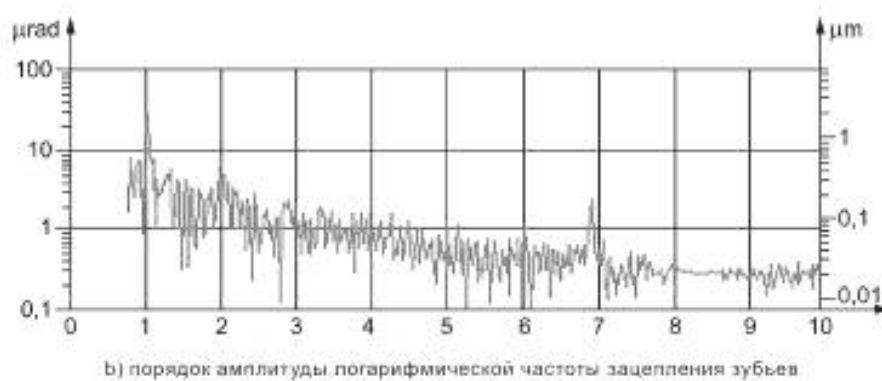
Рисунок F.4, лист 2
