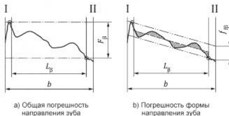
Рисунок 15 — Утолщение зуба при контроле направления зуба
