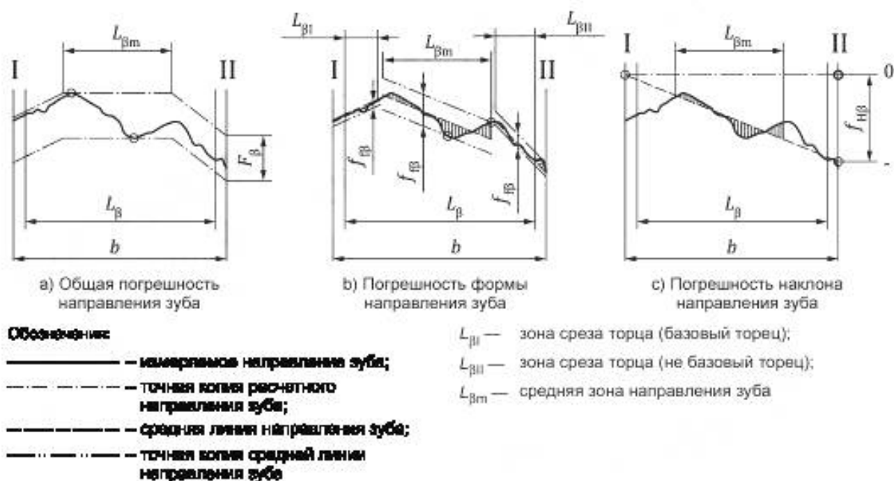
Рисунок А.4 — Контроль направления зуба со срезанными торцами с обеих сторон
