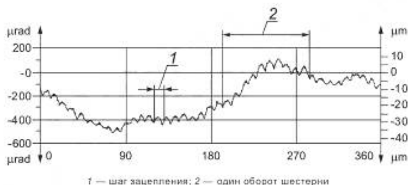
Рисунок F.2 — Пример кинематической погрешности
