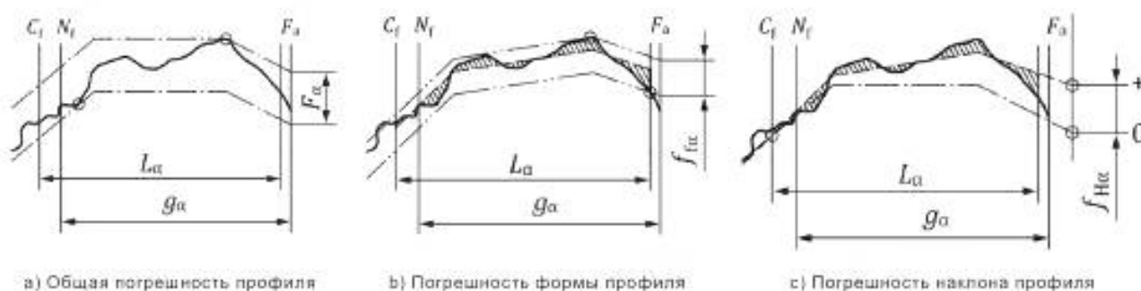
Рисунок 7 — Погрешности профиля с модифицированной головкой
