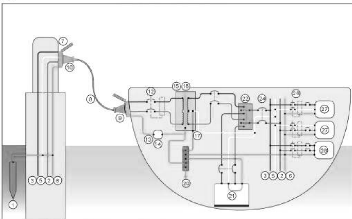
г) Система разделительного трансформатора с однофазным входом 240 В, выходом 120/240 В и генератором, демонстрирующая использование шины заземления основного переменного тока и УЗО/прерывателя берегового питания. Схема приведена с заземленным входом, подсоединенным к системе заземления судна (посредством дополнительного гальванического разъединителя) с преобразованием разъединительного трансформатора в трансформатор полярности.
