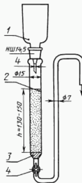
1 — резервуар вместимостью 50 см 3 ; 2 — колонка с каломием; 3 — стекловата; 4 — кран
