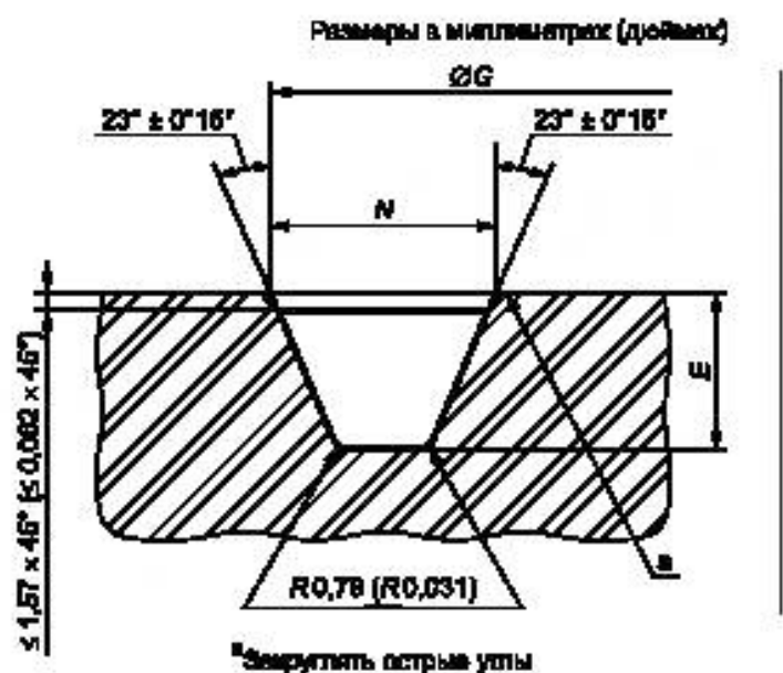
Рисунок 6 — Окончательная механическая обработка кольцевых канавок типа SR
