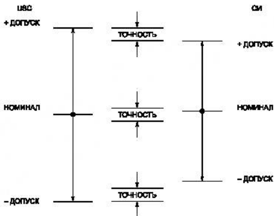
а) Двухсторонний допуск
