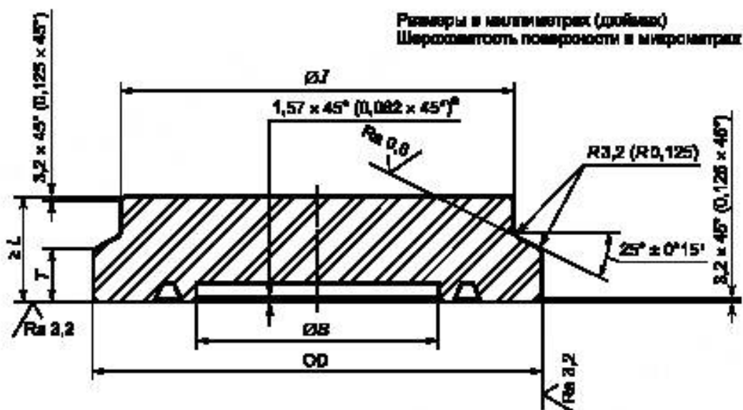
Рисунок 3 — Цельные бугельные соединения типа 16В и 16ВХ
