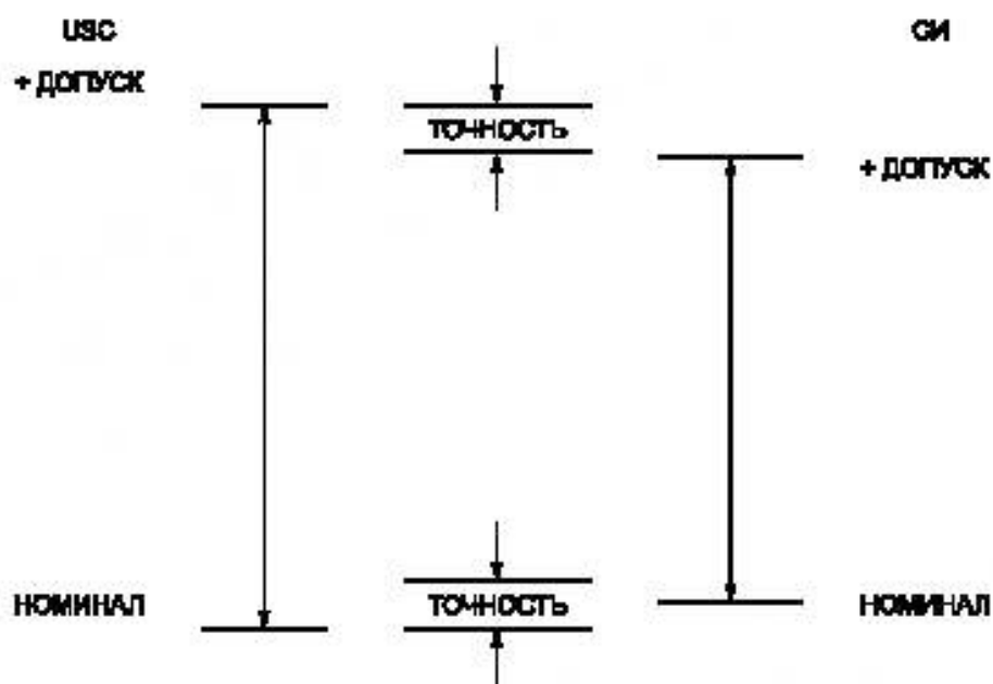
б) Односторонний допуск
