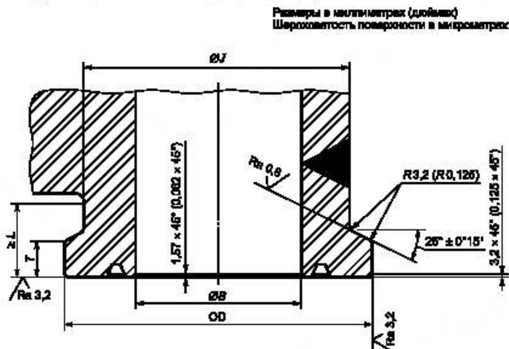
Рисунок 3 — Цельные бугельные соединения типа 16В и 16ВХ
