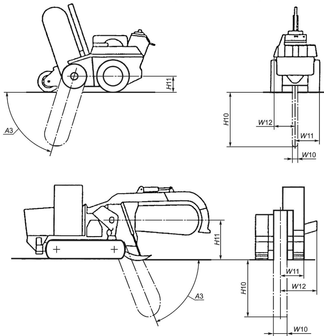
Рисунок 4 — Размеры цепного траншекопателя
