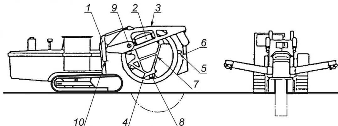
Рисунок 8 — Размеры роторного траншеекопателя
