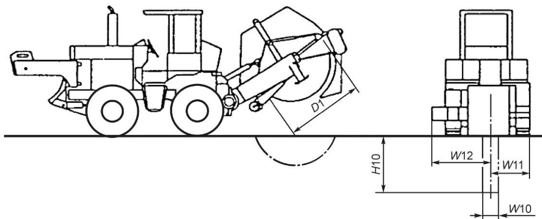
Рисунок 6 — Размеры дискового траншеекопателя
