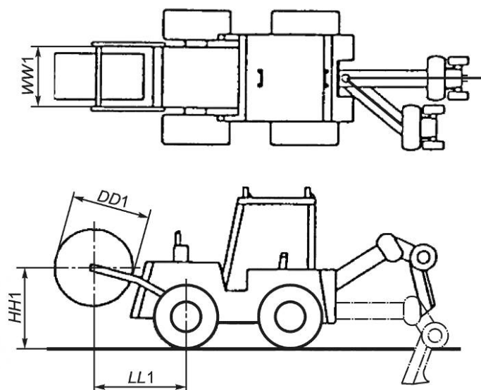
Рисунок 12 — Размеры держателя барабана
