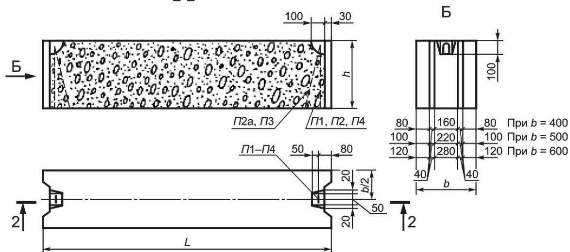
Рисунок 1 — Блоки типа ФБС
