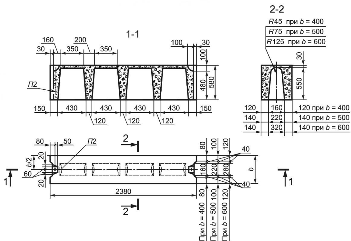
Рисунок 2 — Блоки типа ФБВ
