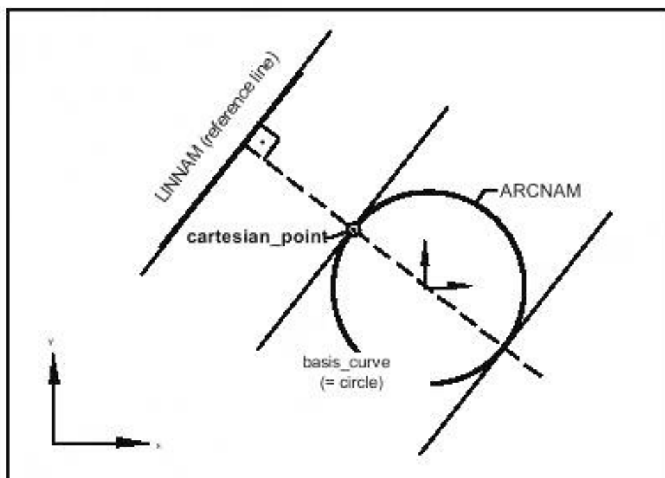
LINNAM (reference line) — ссылочная прямая линия; ARCNAM — дуга окружности; cartesian_point — декартова точка; basis_curve (= circle) — базовая кривая (окружность)
