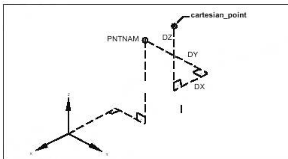
Cartesian_point — результирующая точка; PNTNAM — исходная точка
