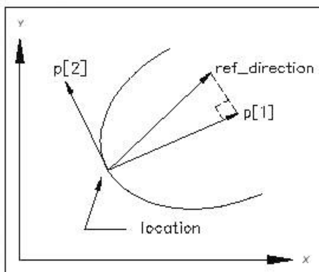
Рисунок 8 — Парабола
