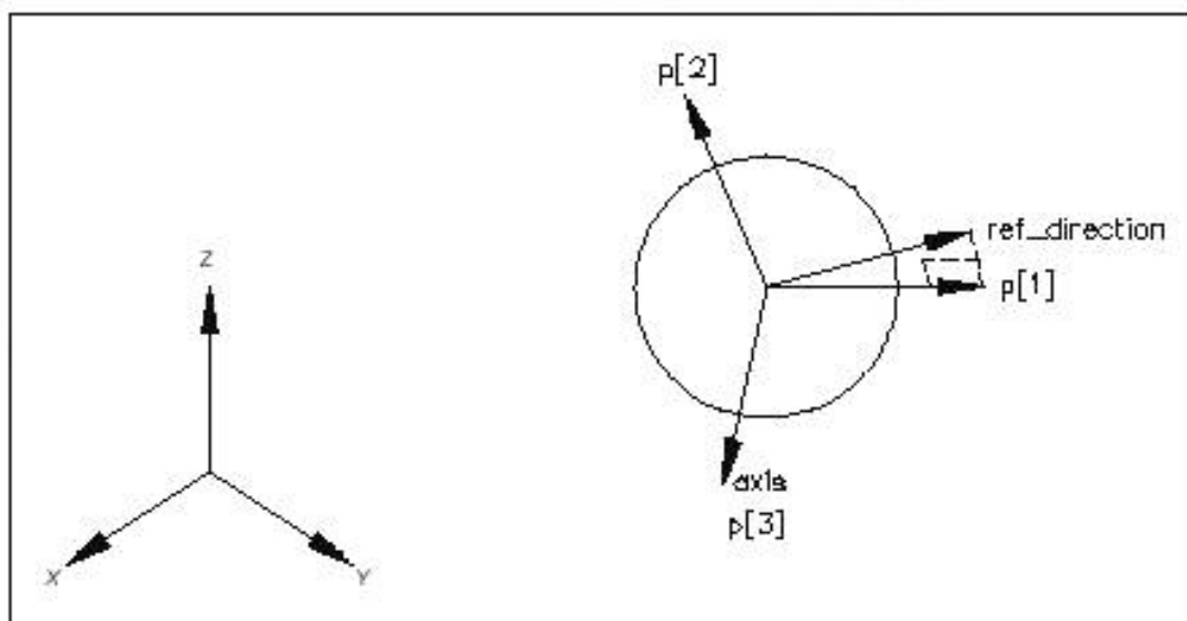
Рисунок 5 — Окружность
