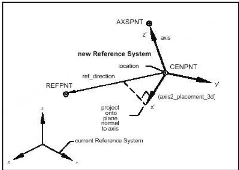
AXSPNT — точка на новой оси Z'; axis — ось; new Reference System — новая ссылочная система; location — начало координат новой системы; CENPNT — точка CENPNT; ref_direction — ссылочное направление; REFPNT — ссылочная точка REFPNT; axis2_placement_3d — локальная координатная система; project onto plane normal to axis — проекция на плоскость, перпендикулярную оси; current Reference System — текущая ссылочная система
