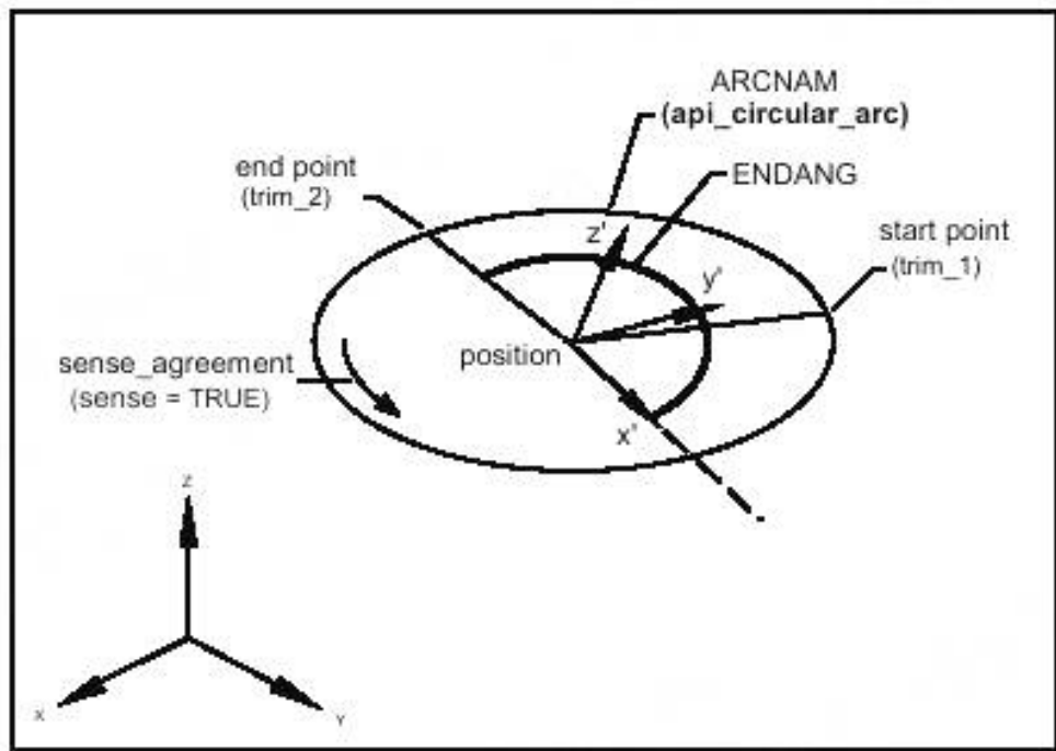
ARCNAME ( api_circular_arc ) — дуга окружности ARCNAM; end point (trim_2) — конечная точка дуги (точка вычленения 2); ENDANG — конечный угол дуги окружности; start point (trim_1) — начальная точка дуги (точка вычленения 1); position — центр окружности; sense_agreement (sense = TRUE) — положительное направление обхода кривой
