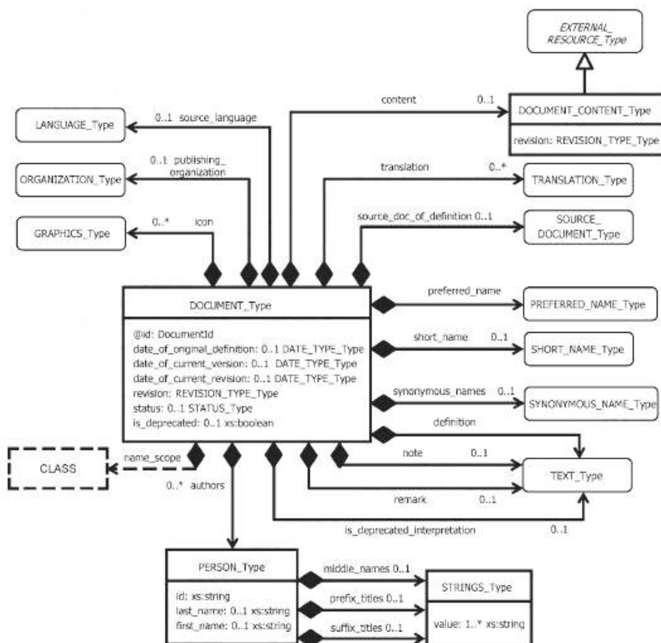
Рисунок 36 — UML-диаграмма документа простого уровня
