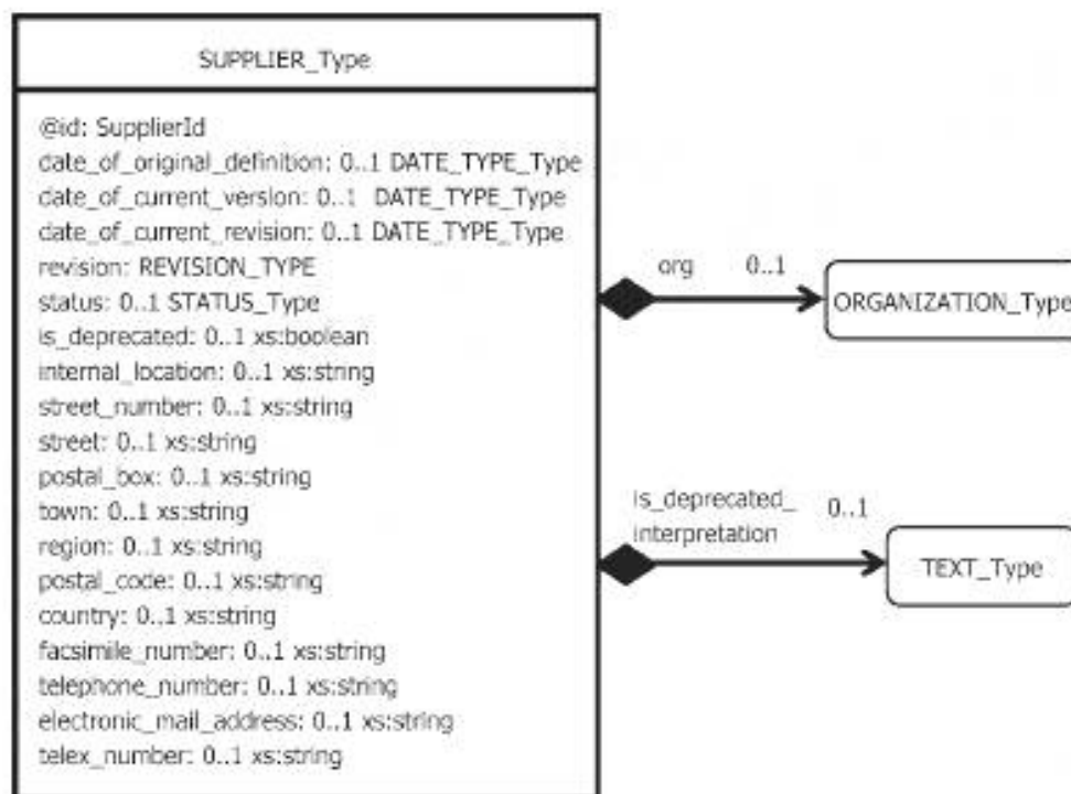
Рисунок 23 — UML-диаграмма онтологии поставщика
