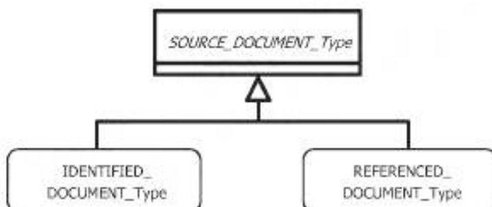
Рисунок 51 — Внешние ресурсы: Документы — источники информации
