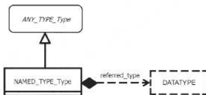
Рисунок 73 — Структура именованного типа данных
