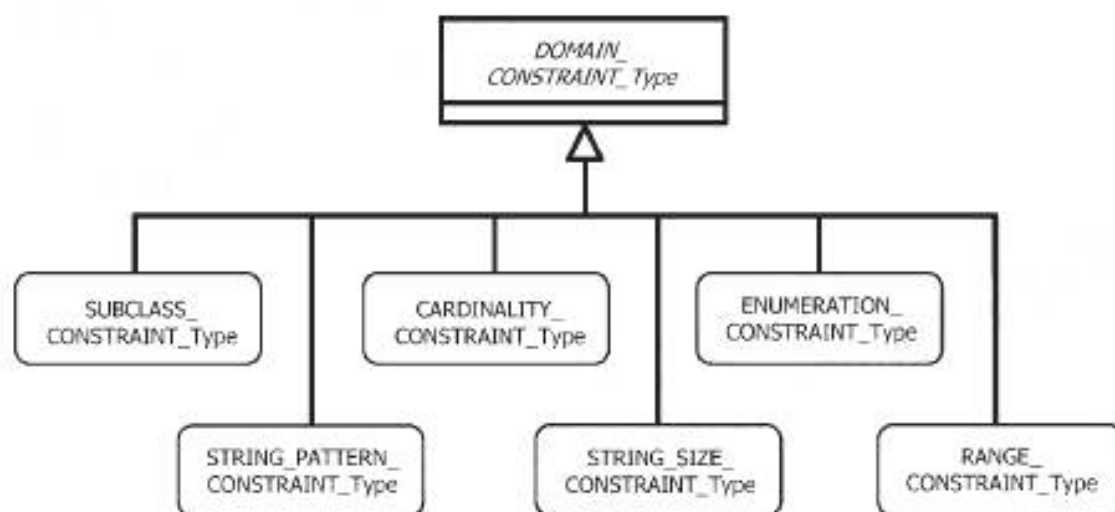
Рисунок 91 — Структура ограничительного условия на область значений
