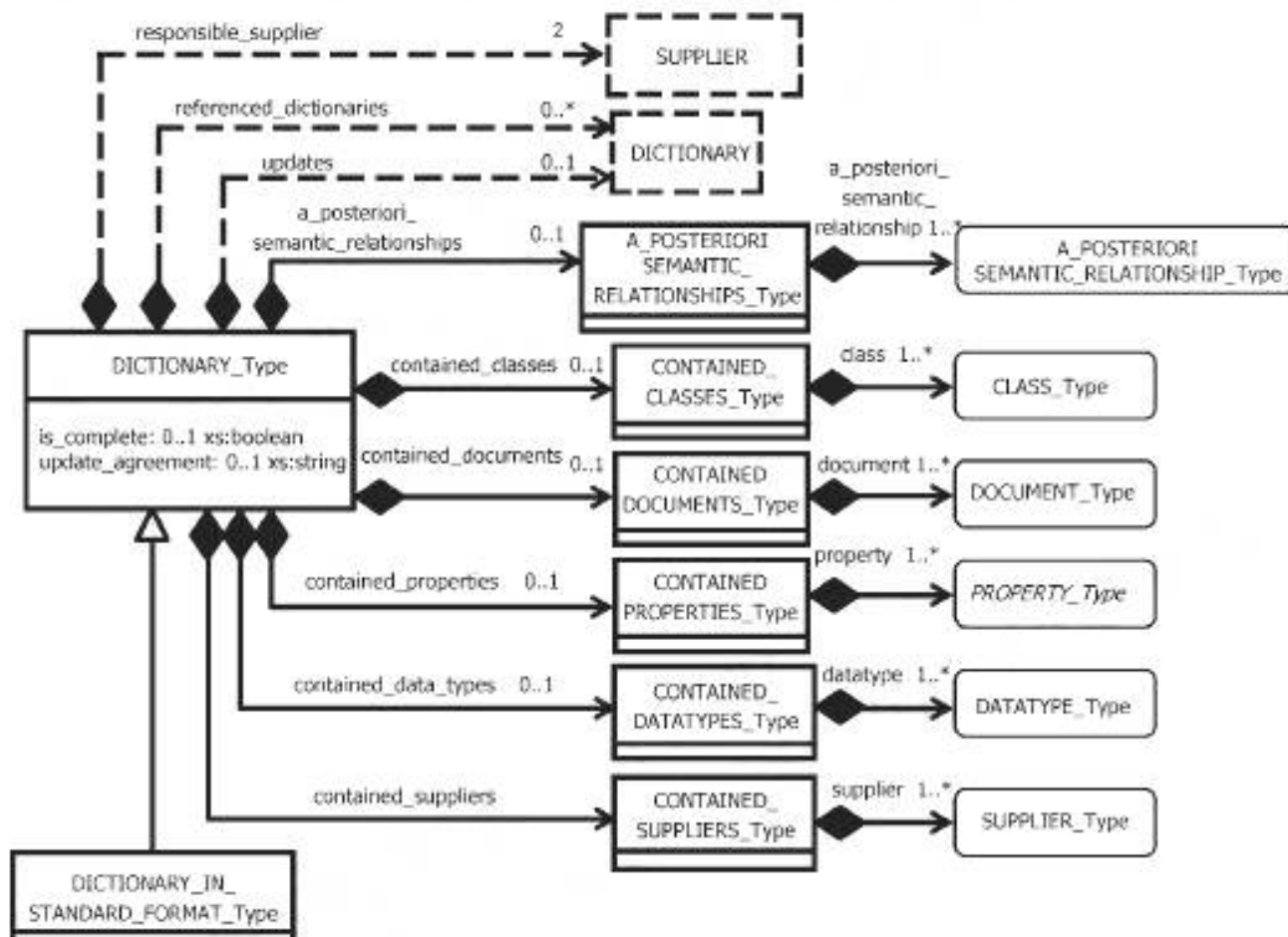
Рисунок 22 — Корневой элемент онтологии
