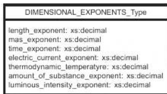
Рисунок 78 — Структура показателя размерности
