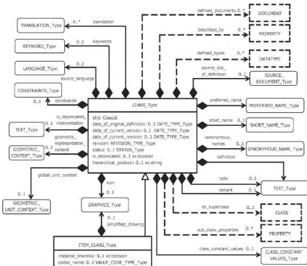
Рисунок 24 — UML-диаграмма, иллюстрирующая понятие простого класса онтологии
