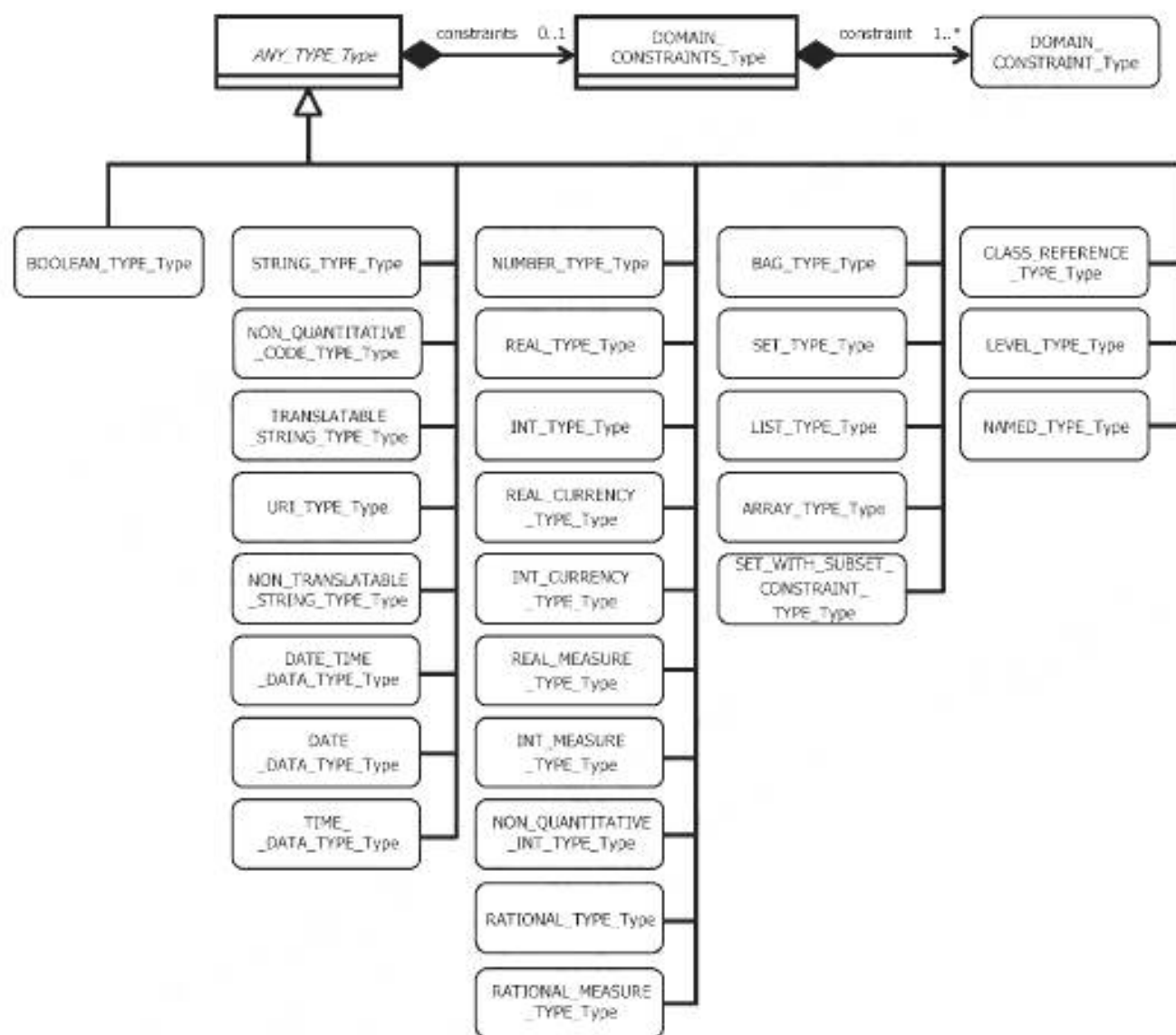
Рисунок 57 — OntoML-система типов данных
