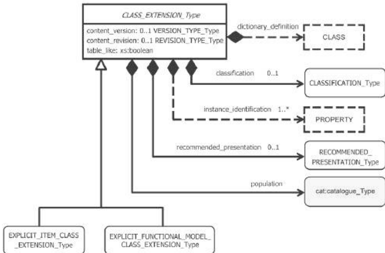
Рисунок 38 — Обобщенная структура класса расширения
