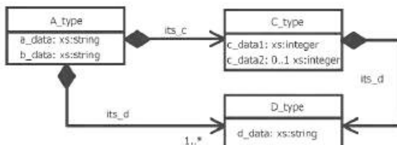
Рисунок F.2 — UML-подобное представление информационной модели
