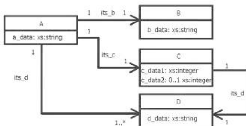
Рисунок F.1 — Пример информационной UML-модели
