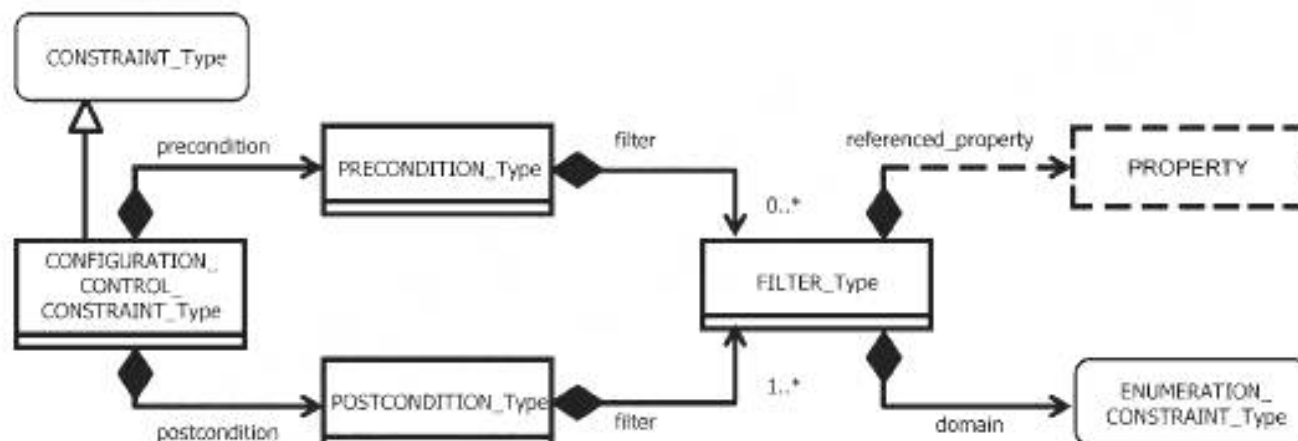
Рисунок 87 — Структура ограничительного условия на управление конфигурацией
