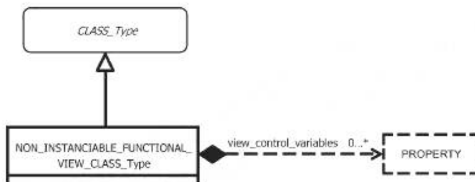
Рисунок 29 — UML-диаграмма понятия класса в онтологии повышенного уровня
