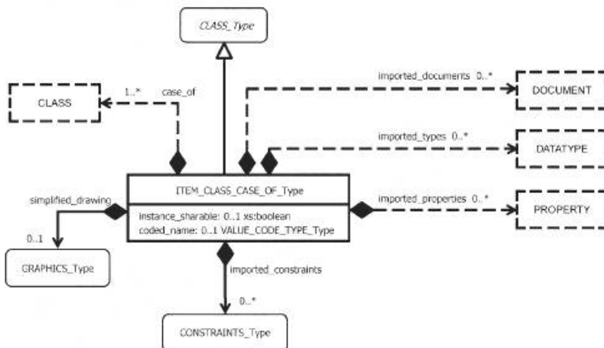
Рисунок 27 — UML-диаграмма условного класса элементов
