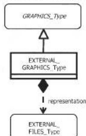
Рисунок 55 — Внешние ресурсы: Внешние графические материалы
