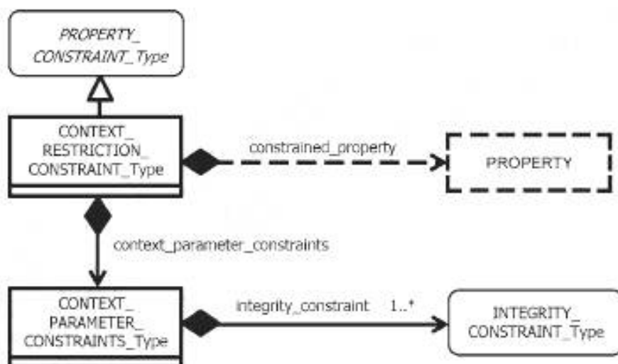
Рисунок 89 — Структура ограничительного условия на контекст
