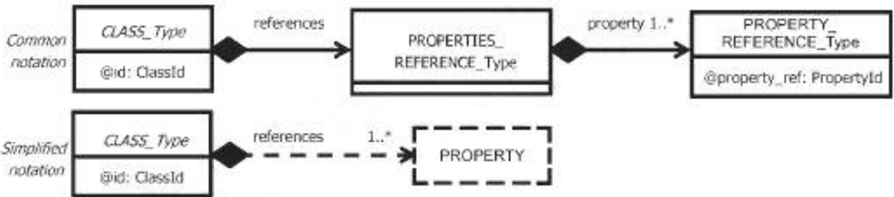
Рисунок 18 — UML-представление многозначной ссылки между понятиями CIIM-онтологии
