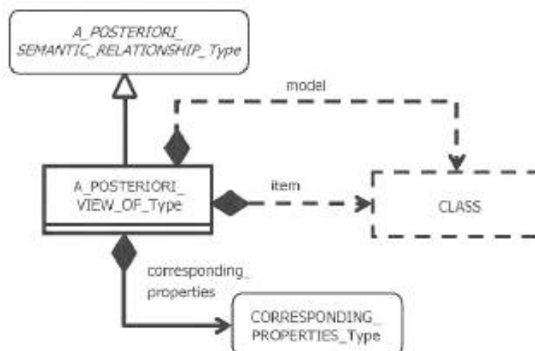
Рисунок 100 — Структура апостериорного производного семантического отношения
