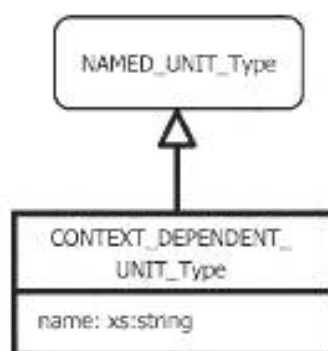
Рисунок 82 — Структура контекстно-зависимой единицы измерений
