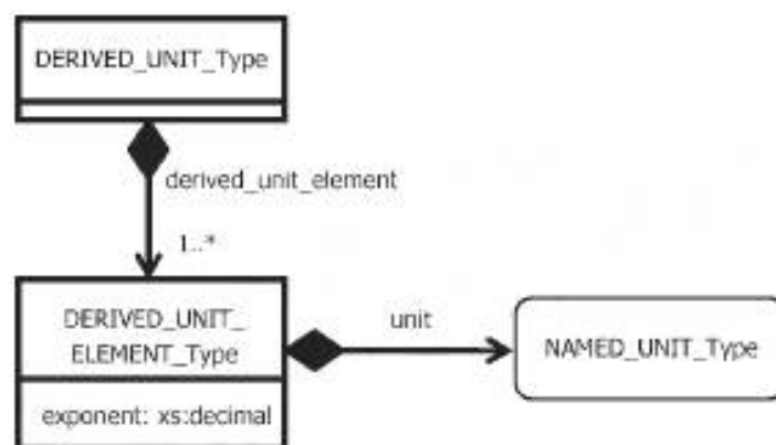
Рисунок 83 — Структура производной единицы измерений
