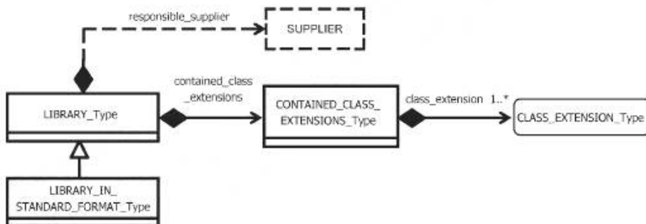
Рисунок 37 — Корневой элемент библиотеки
