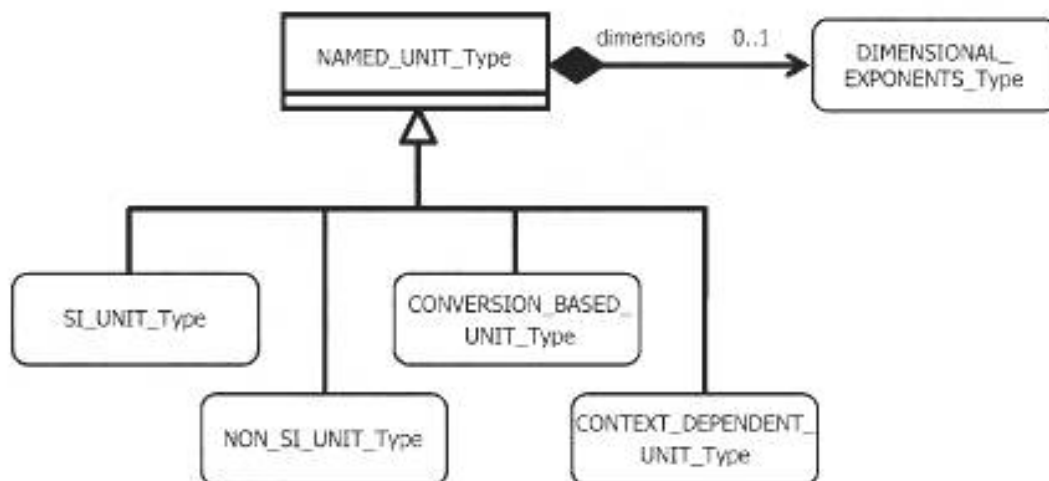
Рисунок 77 — Общая структура именованных единиц измерений
