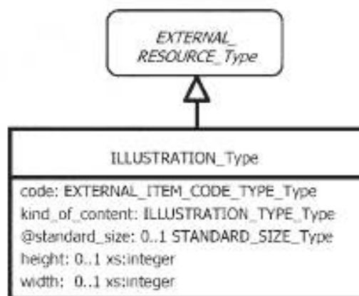
Рисунок 48 — Онтология элементарного уровня для внешних ресурсов: Иллюстрация
