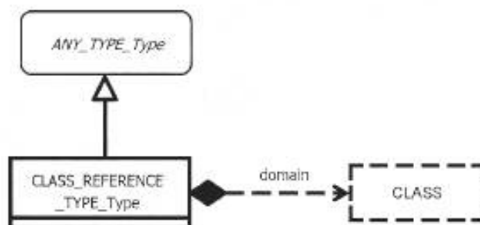
Рисунок 71 — Структура области значений экземпляра класса
