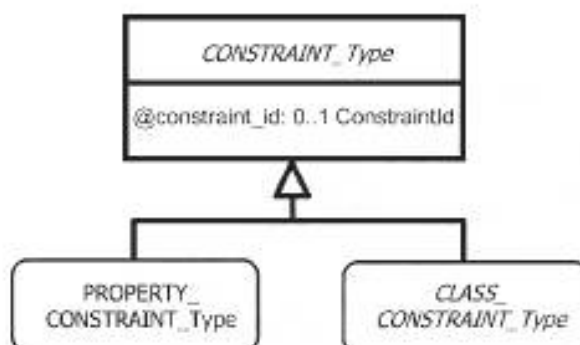
Рисунок 84 — Общая структура ограничительных условий
