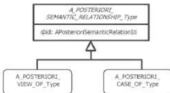
Рисунок 98 — Структура апостериорного семантического соотношения
