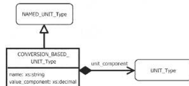
Рисунок 81 — Структура преобразованной единицы измерений
