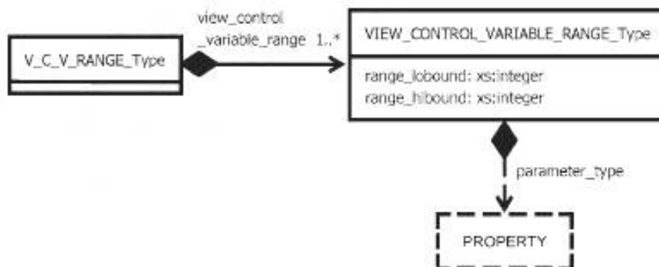
Рисунок 32 — Структура контрольной переменной представления
