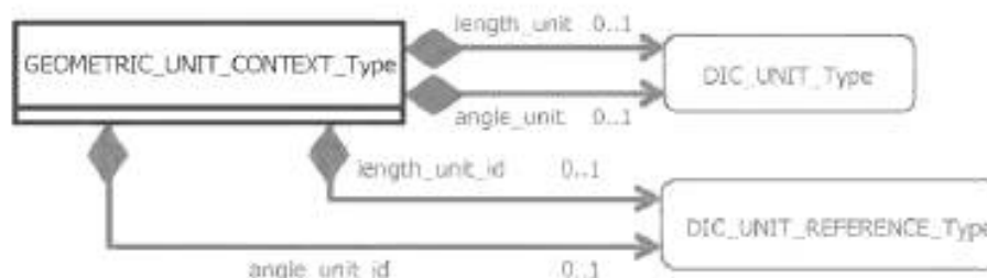
Рисунок 106 — Структура единицы измерения геометрического контекста
