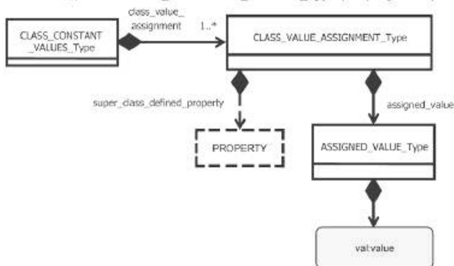
Рисунок 28 — Структура присвоенного значения класса
