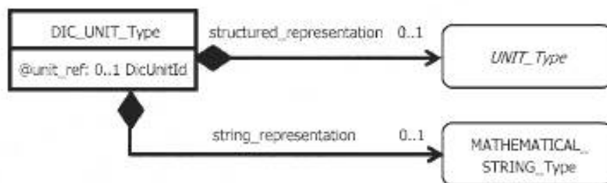
Рисунок 75 — Общая структура единиц измерения свойства
