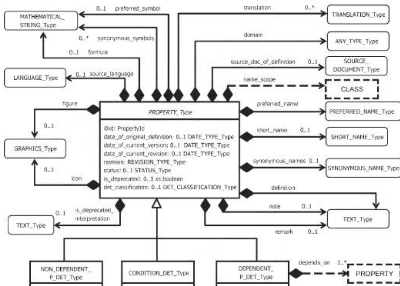
Рисунок 33 — UML-диаграмма понятия простого онтологического свойства
