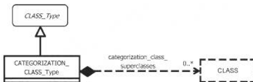
Рисунок 26 — Класс категоризации
