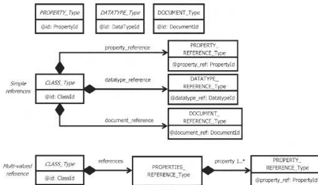
Рисунок 15 — Ссылка на понятие CIIM-онтологии
