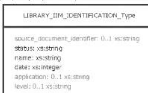
Рисунок 101 — Структура идентификации, интегрированной в библиотеку информационной модели
