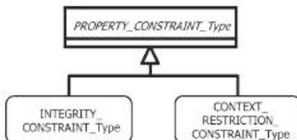
Рисунок 88 — Структура ограничительного условия на свойство
