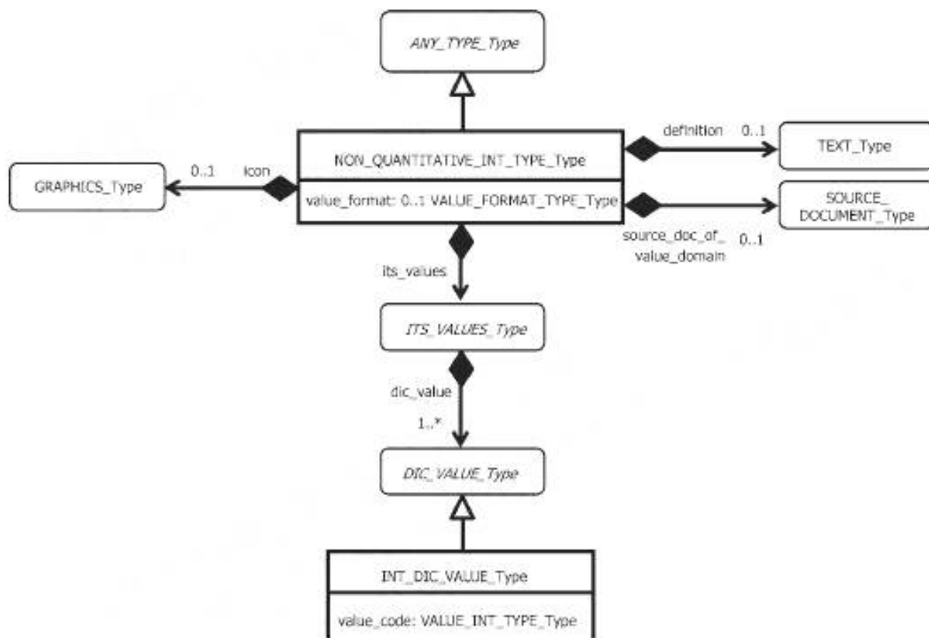
Рисунок 65 — Структура перечня типов целочисленных кодов
