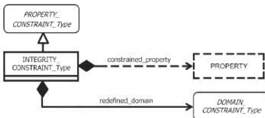
Рисунок 90 — Структура ограничительного условия на целостность данных
