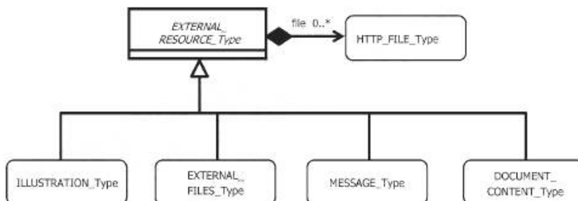
Рисунок 46 — Онтология элементарного уровня для внешних ресурсов
