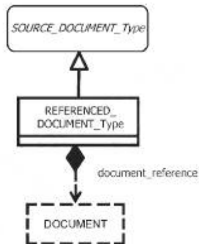
Рисунок 53 — Внешние ресурсы: Ссылочный документ
