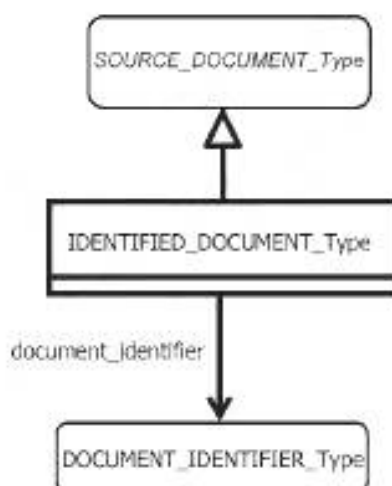
Рисунок 52 — Внешние ресурсы: Идентифицированный документ
