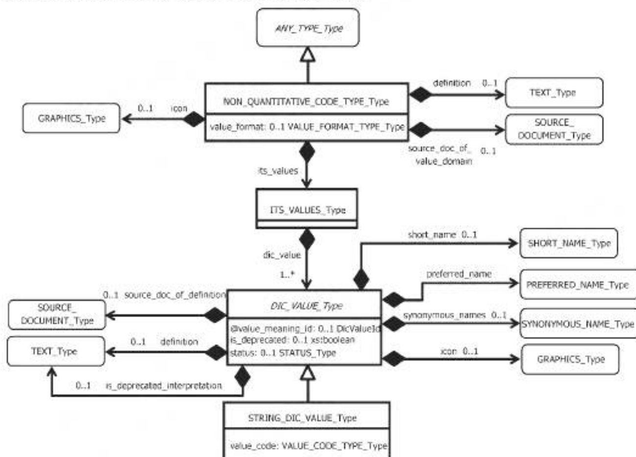
Рисунок 61 — Структура типа перечислимых строковых кодов
