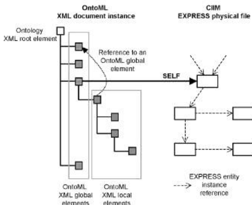
Рисунок F.6 — Глобальные и локальные XML-элементы
