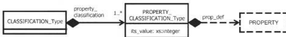
Рисунок 39 — Классификация свойств
