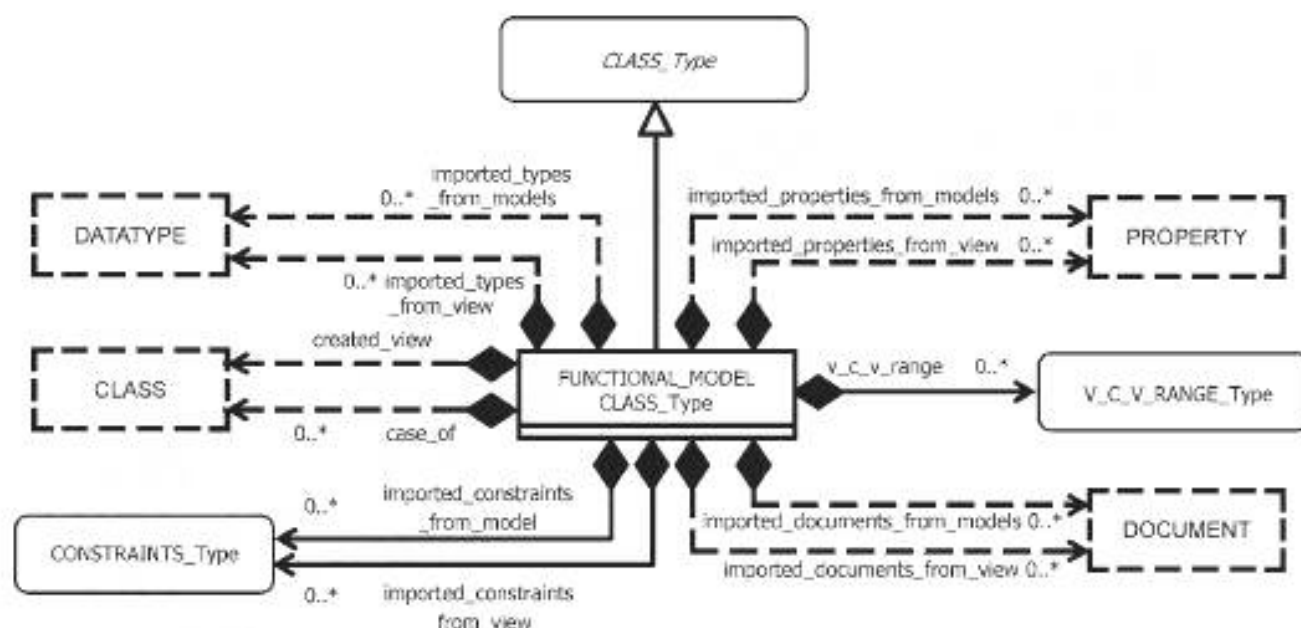
Рисунок 30 — UML-диаграмма онтологического понятия повышенного класса
