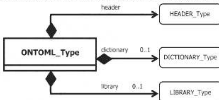
Рисунок 20 — UML-диаграмма структуры онтологии
