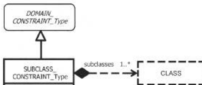
Рисунок 92 — Структура ограничительного условия на подкласс
