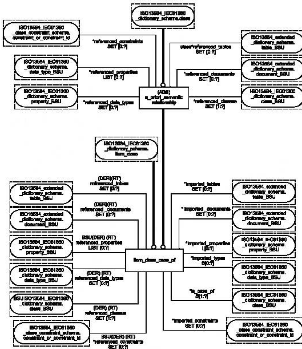
Рисунок 1.10 — Диаграмма EXPRESS-G № 1 (единственная) для стандартной схемы условного класса продуктов ISO13584_IEC61360_item_class_case_of_schema
