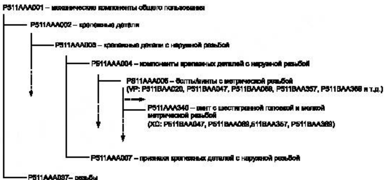
Рисунок 4 — Месторасположение и некоторые унаследованные свойства класса P511AAA340
