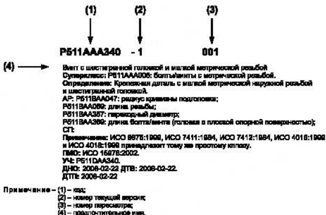
Рисунок 3 — Раскладка определения класса
