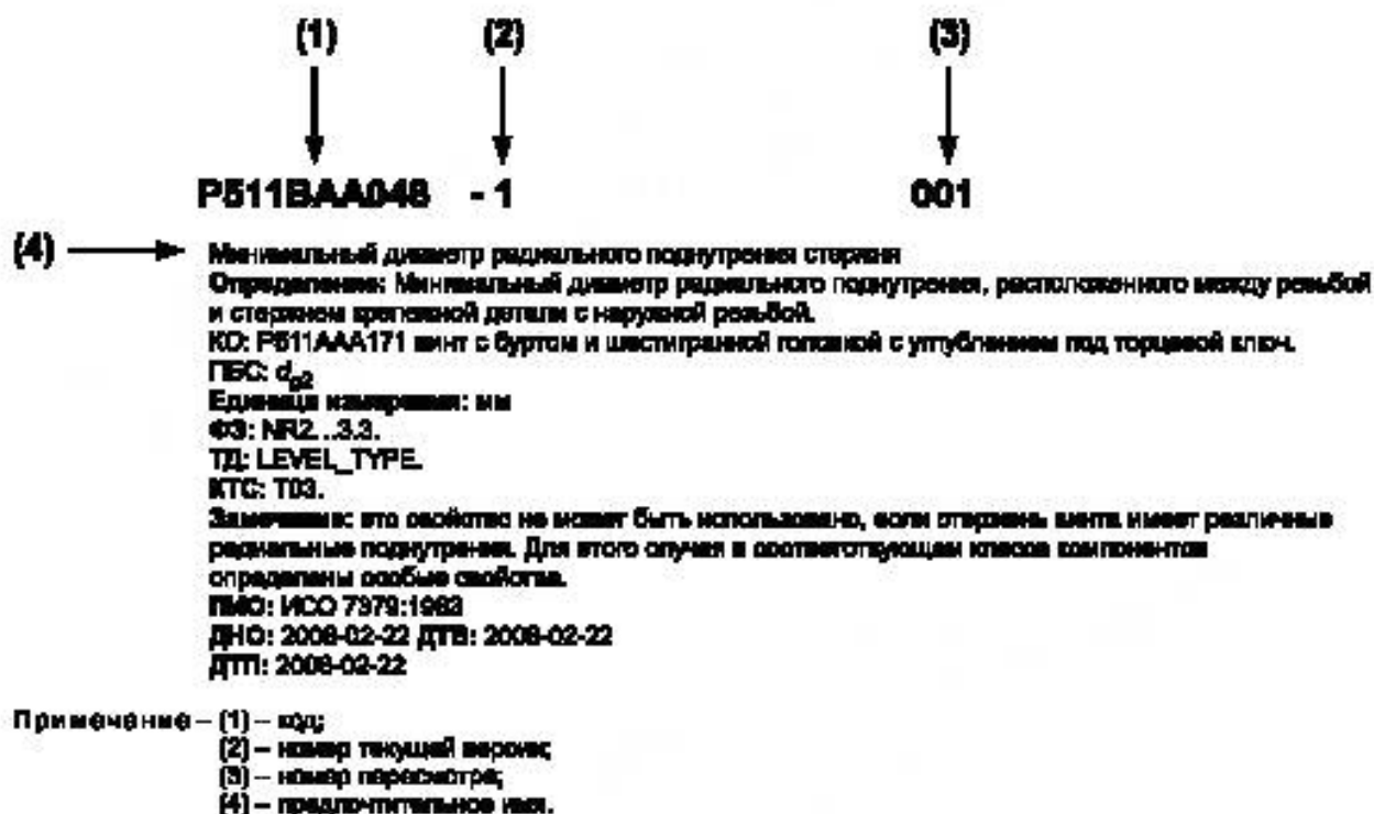
Рисунок 5 — Раскладка определения ТЭД свойств
