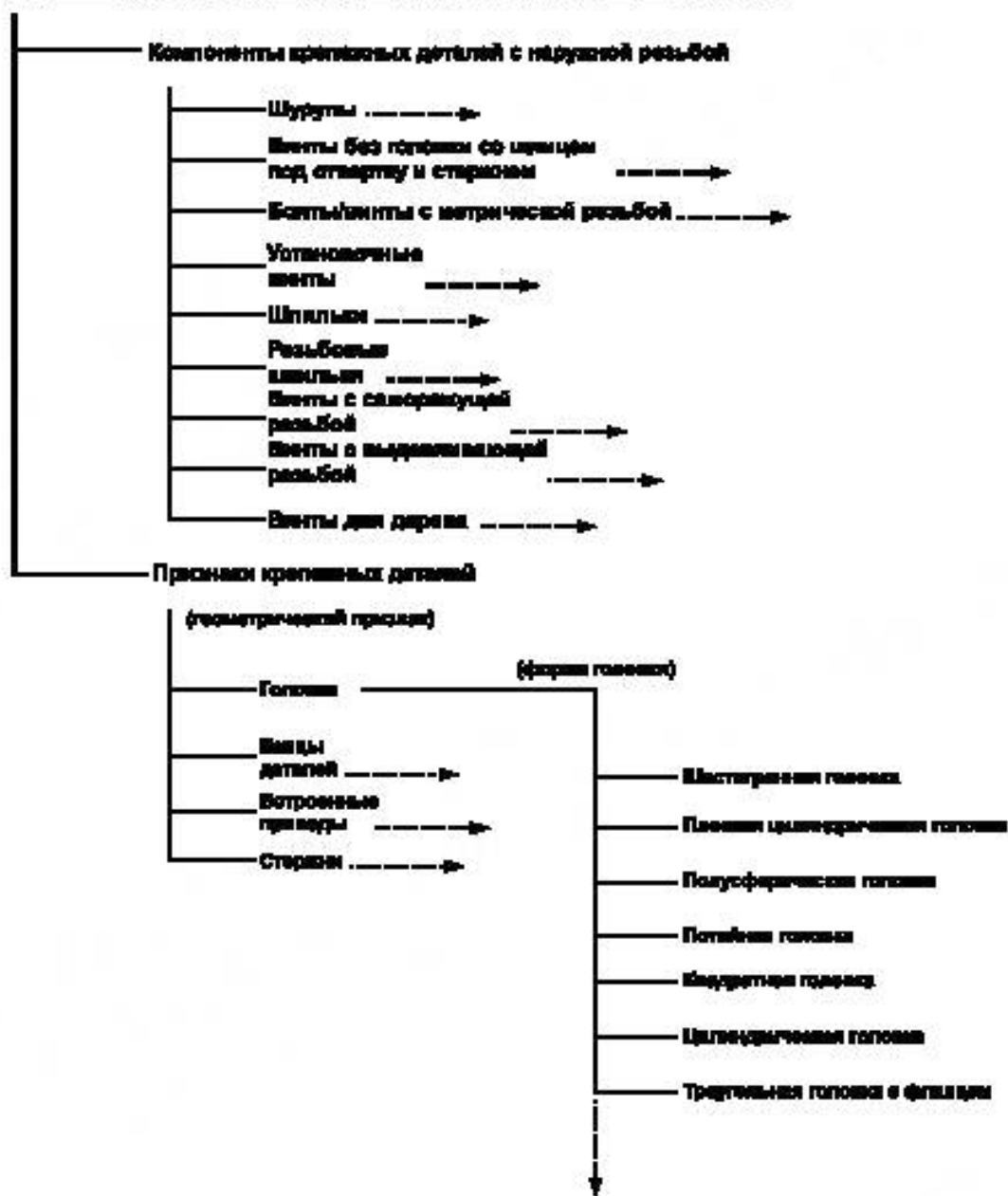
Рисунок 2 — Структура класса крепежные детали с наружной резьбой
