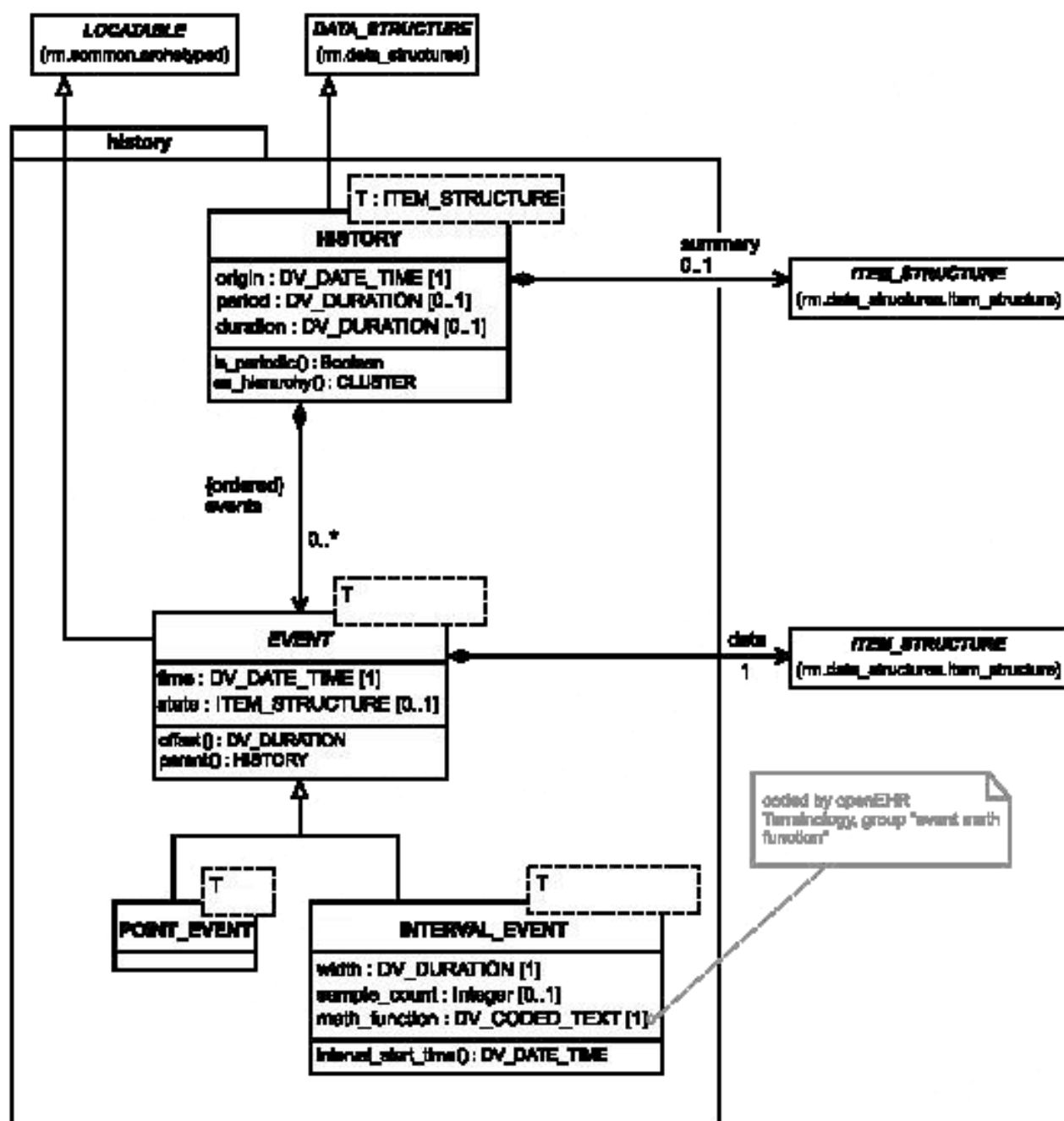
Рисунок А.3 — Пакет HISTORY openEHR
