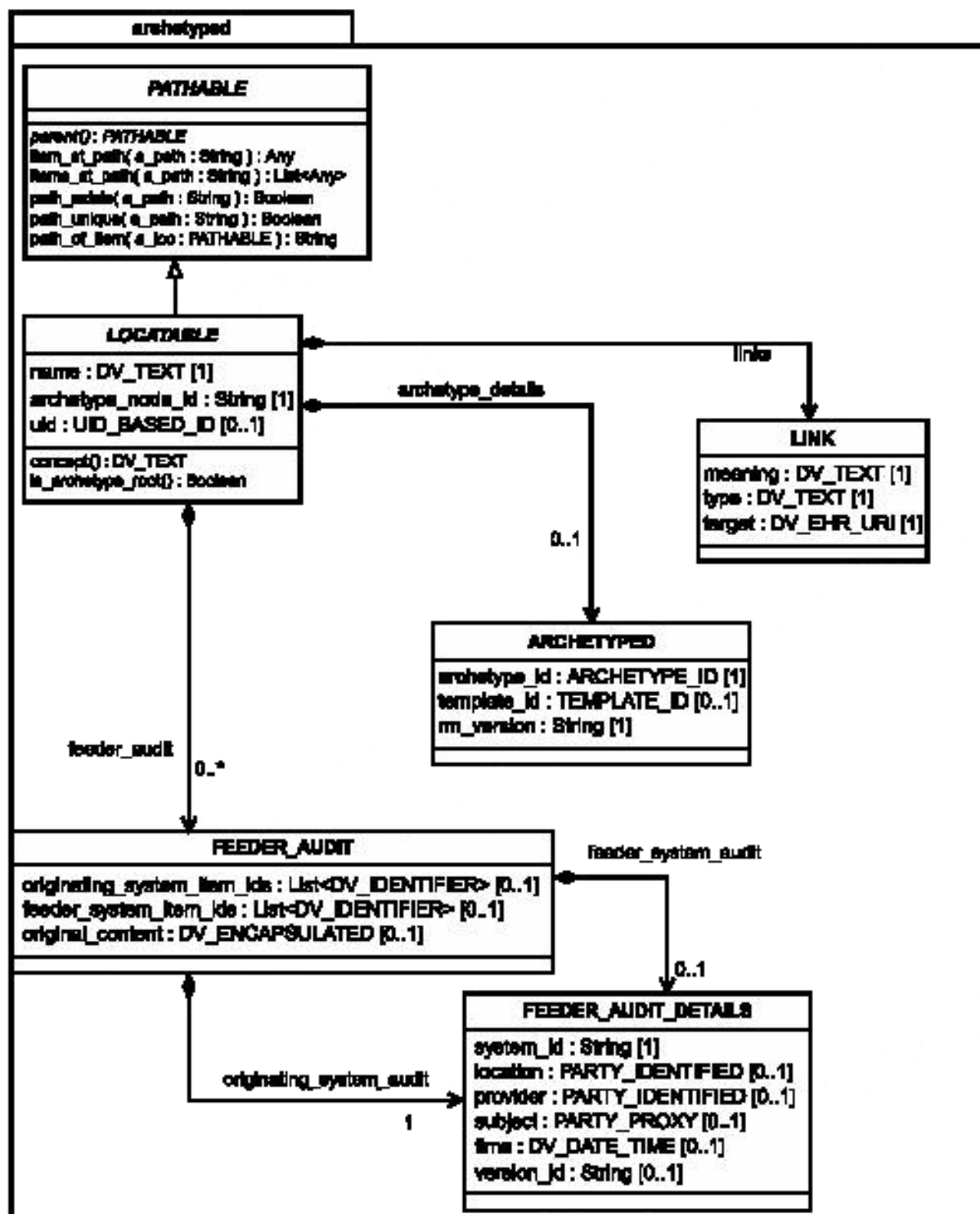
Рисунок А.1 — Пакет архетипов opelEHR
