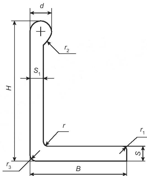
Рисунок 1 — Прессованный бульбообразный профиль углового сечения
