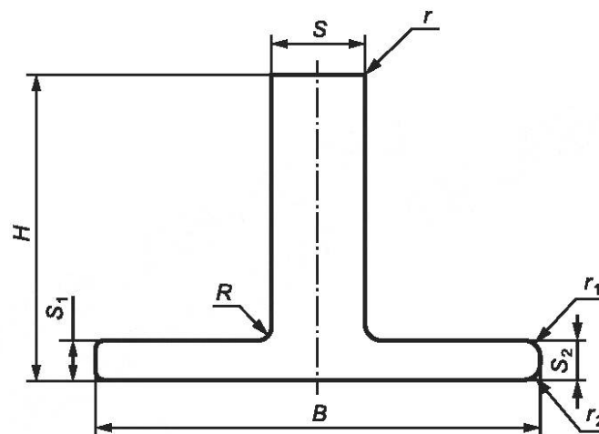
B — длина; H — высота; S , S_1 , S_2 — толщина; r , r_1 , r_2 — радиусы притупления; R — радиус скругления Рисунок 1 — Прессованный прямоугольный профиль равнополочного таврового сечения
