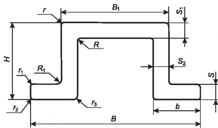
Рисунок 1 — Прессованный прямоугольный профиль отбортованного швеллерного сечения
