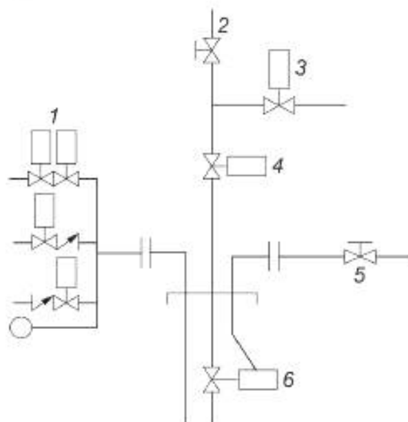
1 — CID; 2 — PSV; 3 — PWV; 4 — PMV; 5 — изоляция SCSSV; 6 — SCSSV
