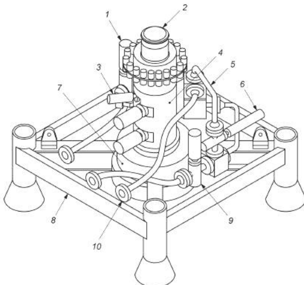
1 — эксплуатационная боковая задвижка; 2 — заглушка устьевой елки; 3 — эксплуатационная коронная задвижка; 4 — блок коренной задвижки; 5 — трубная петля; 6 — перепускная задвижка; 7 — соединитель устьевой елки; 8 — направляющая рама устьевой елки; 9 — боковая задвижка канала кольцевого пространства; 10 — соединитель выкидного трубопровода (выкидной линии)
