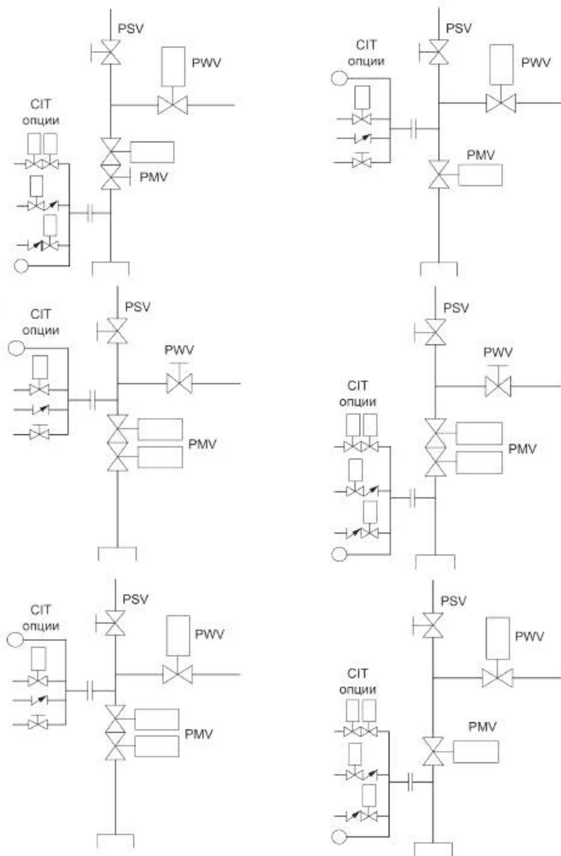
а) Примеры проходок (пенетраций) эксплуатационных каналов
