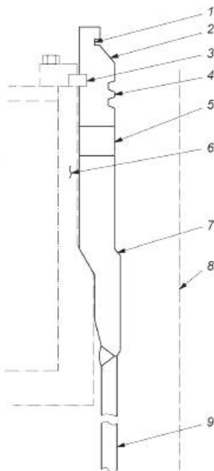
1 — запыление устьевого оголовка; 2 — посадочный заплечик для устьевого оголовка; 3 — крепление постоянной донной направляющей плиты; 4 — подготовка спуско-подъемного инструмента и соединителя колонны-надставки; 5 — цементный порт (опционально); 6 — постоянная донная направляющая плита; 7 — посадочный заплечик; 8 — осевая линия; 9 — кондукторная обсадная колонна
