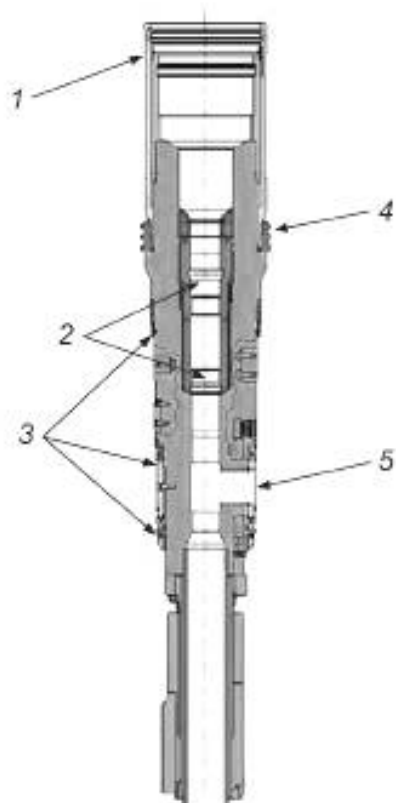
Рисунок D.4 — Трубодержатель НКТ расширенной конфигурации устьевой вилки горизонтального типа
