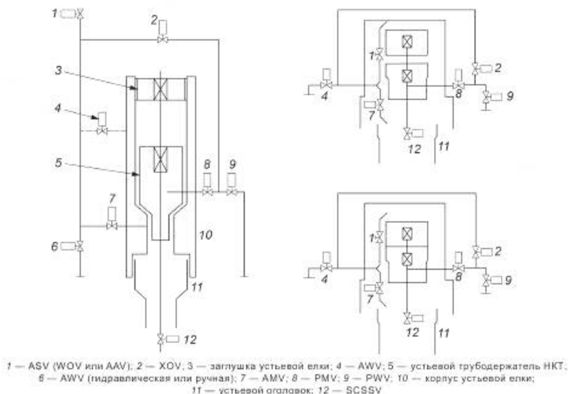
Рисунок 3 — Примеры устьевых елок горизонтального типа
