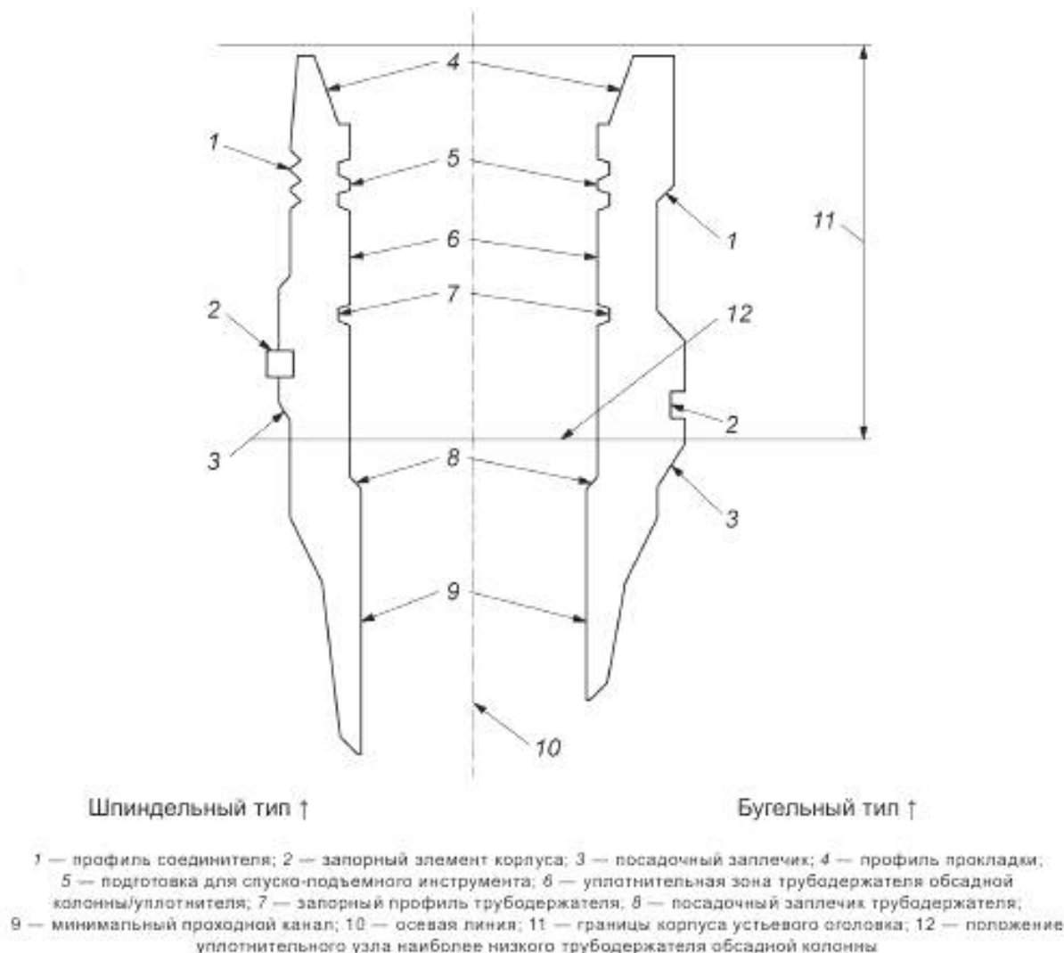
Рисунок 14 — Типовые корпуса устьевых оголовков
