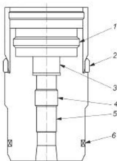
1 — канавка фиксатора спуско-подъемного инструмента; 2 — запорный элемент; 3 — изолирующие карманы стыковочных устройств; 4 — профиль канатной пробки; 5 — эксплуатационный канал; 6 — уплотнение
