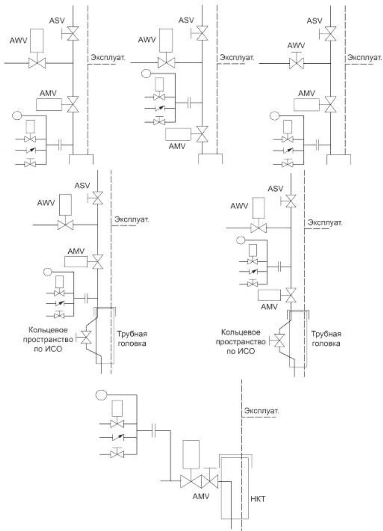
b) Примеры проходов (пенетраций) кольцевых каналов
