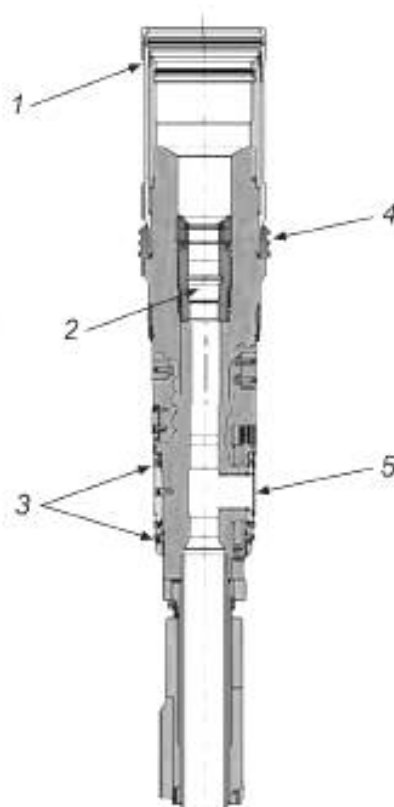
Рисунок D.2 — Трубодержатель НКТ с несколькими проходными каналами
