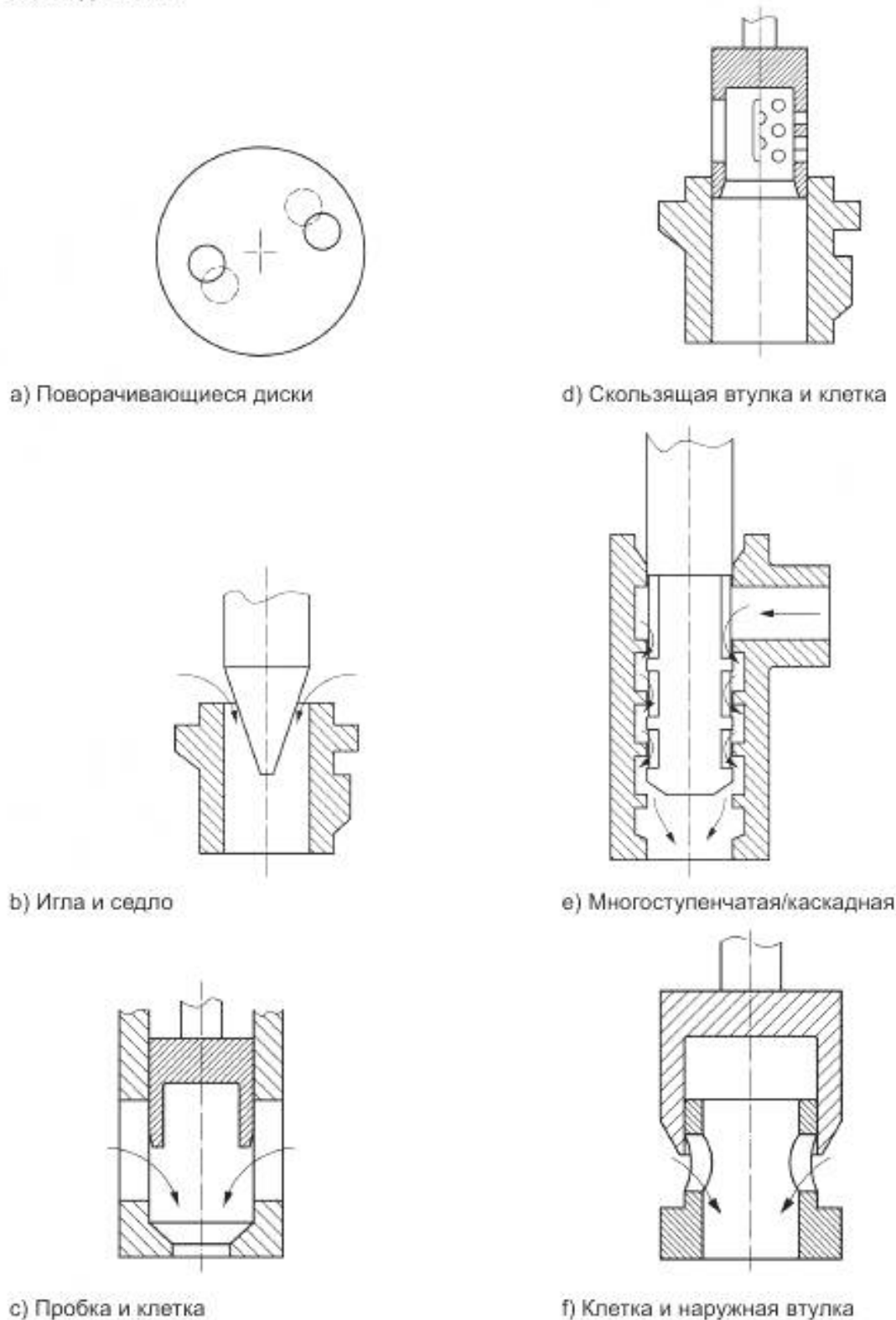
Рисунок 10 — Широко применяемые конфигурации диафрагм дросселя
