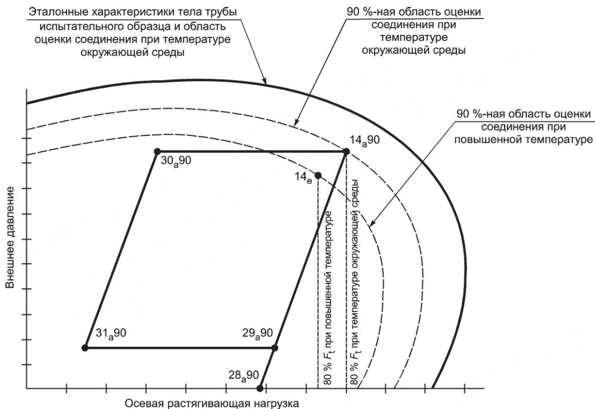
Рисунок 34 — Процедура расчета траектории нагрузки при проведении TS-C
