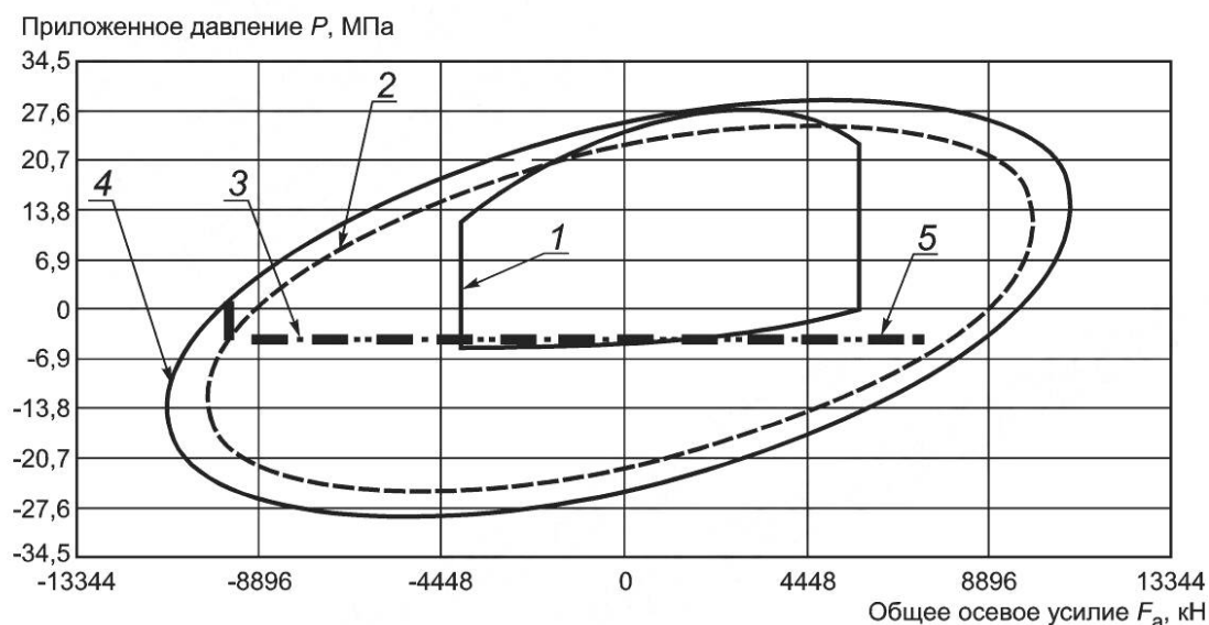
Рисунок D.39 — CEE a испытательного образца
