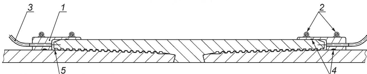
1 — гибкий шланг; 2 — хомуты для шланга; 3 — металлическая трубка или гибкий шланг [термостойкая(ий) для испытаний при повышенной температуре]; 4 — уплотнительный материал; 5 — небольшой зазор для повышения чувствительности выявления утечек
