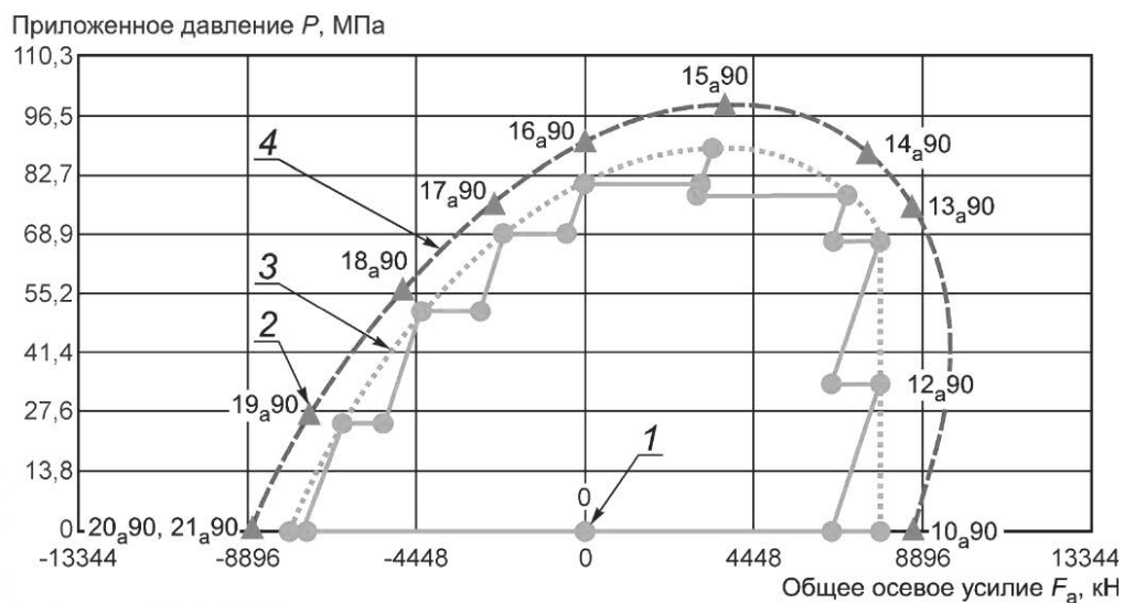
Рисунок D.30 — A a 90 % (QI, QII), TS-A этапы нагрузки 126—148
