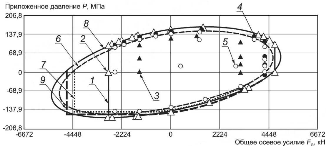
Рисунок D.37 — Точки CEE a и точки нагрузки TLE a
