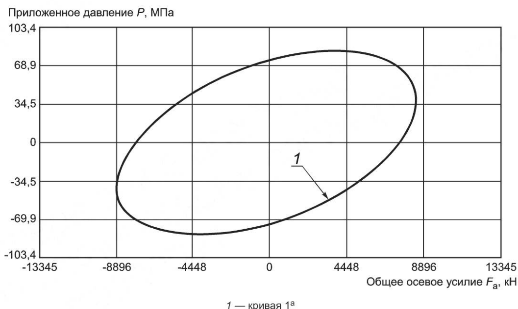
Рисунок D.4 — Кривая 1 а номинального VME тела трубы при температуре окружающей среды
