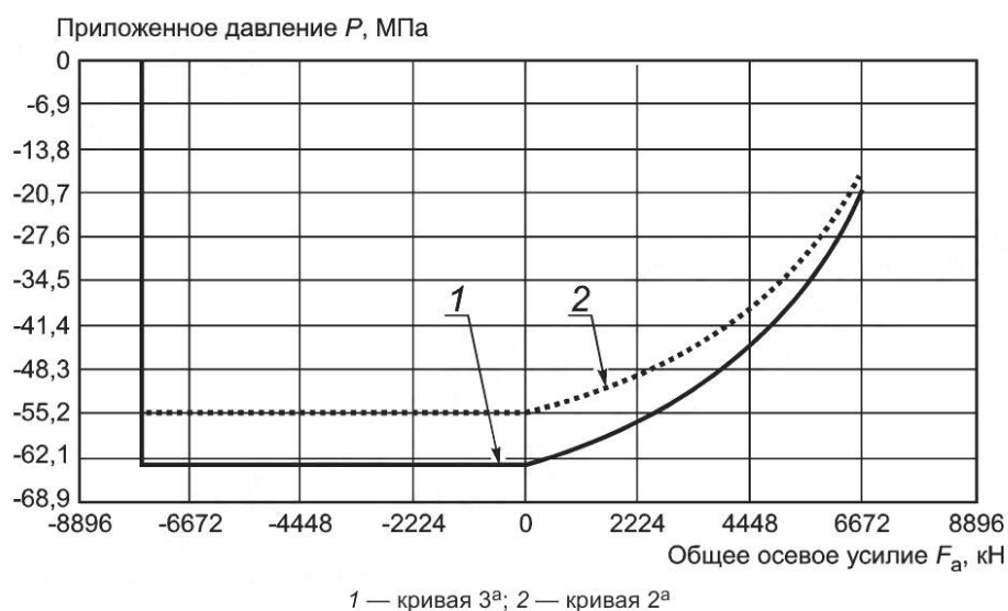
Рисунок D.6 — Кривые номинального давления смятия по API тела трубы 2 a и наружного давления для труб, стойких к смятию 3 a , при температуре окружающей среды
