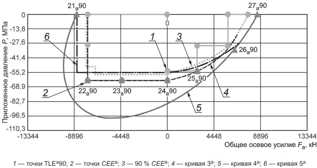
1 — точки TLE a 90; 2 — точки CEE a ; 3 — 90 % CEE a ; 4 — кривая 3 a ; 5 — кривая 4 a ; 6 — кривая 5 a Рисунок D.31 — A a 90 % (QIII, QIV) и A a 90 % (QIV, QIII), TS-A этапы нагрузки 149—175
