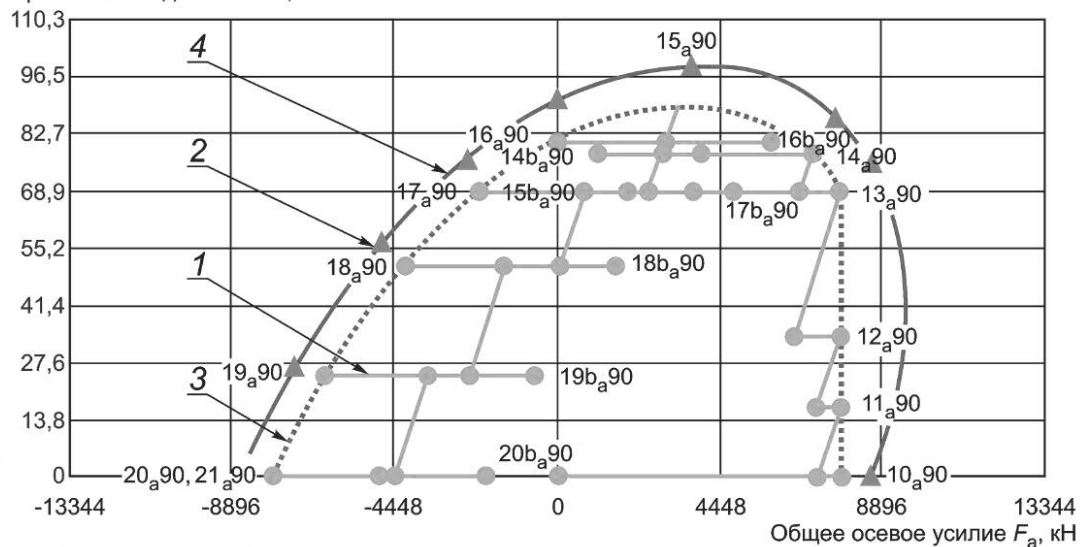
Рисунок D.23 — B^a_b 90 % (QI, QII, QI), TS-B этапы нагрузки 156—244
