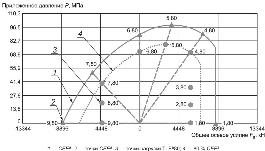
Рисунок D.16 — Точки CEE^a и точки нагрузки 80 % TLE^a при температуре окружающей среды
