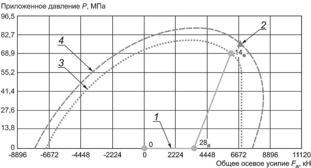
1 — точки TLE e ; 2 — точки CEE e ; 3 — 90 % CEE e ; 4 — кривая 4 e Рисунок D.24 — Десять термических циклов, TS-C этапы нагрузки 1—44
