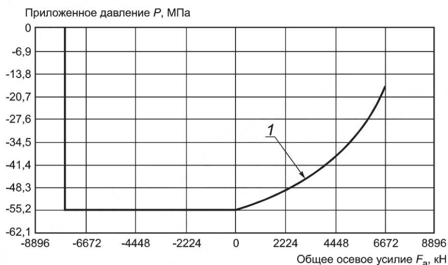
1 — кривая 2 а
