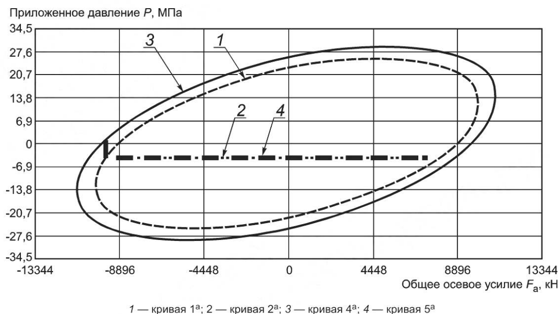
Рисунок D.38 — Эталонные характеристики испытательного образца тела трубы (кривые 1 a , 2 a , 4 a и 5 a )
