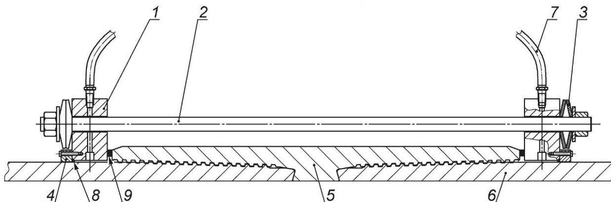
1 — металлический фланец; 2 — резьбовая шпилька; 3 — пружины; 4 — резьбовая гайка; 5 — муфта; 6 — труба; 7 — гибкий шланг (термостойкий для испытаний при повышенной температуре); 8 — уплотнительное кольцо; 9 — прокладка с гладкой поверхностью
