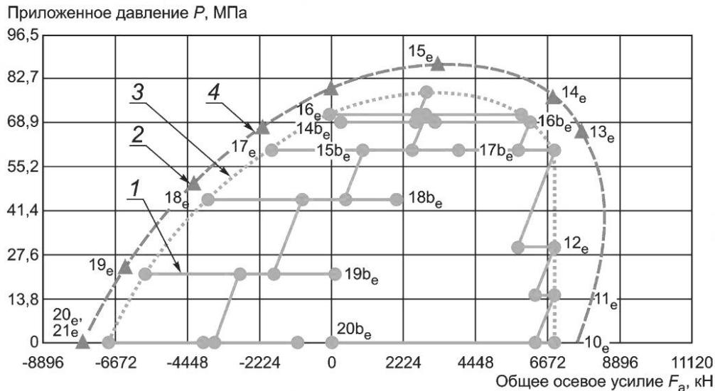
Рисунок D.22 — B e 90 % (QI, QII, QI), TS-B этапы нагрузки 67—155
