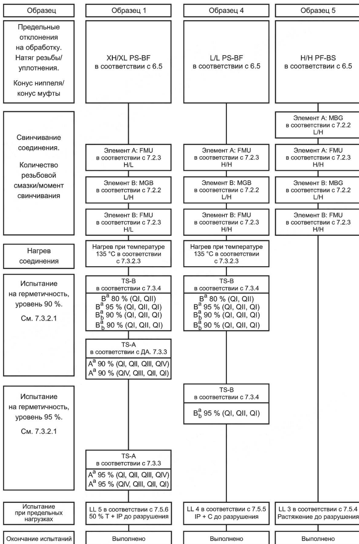
Рисунок 5 — Требования и порядок испытаний при CAL II
