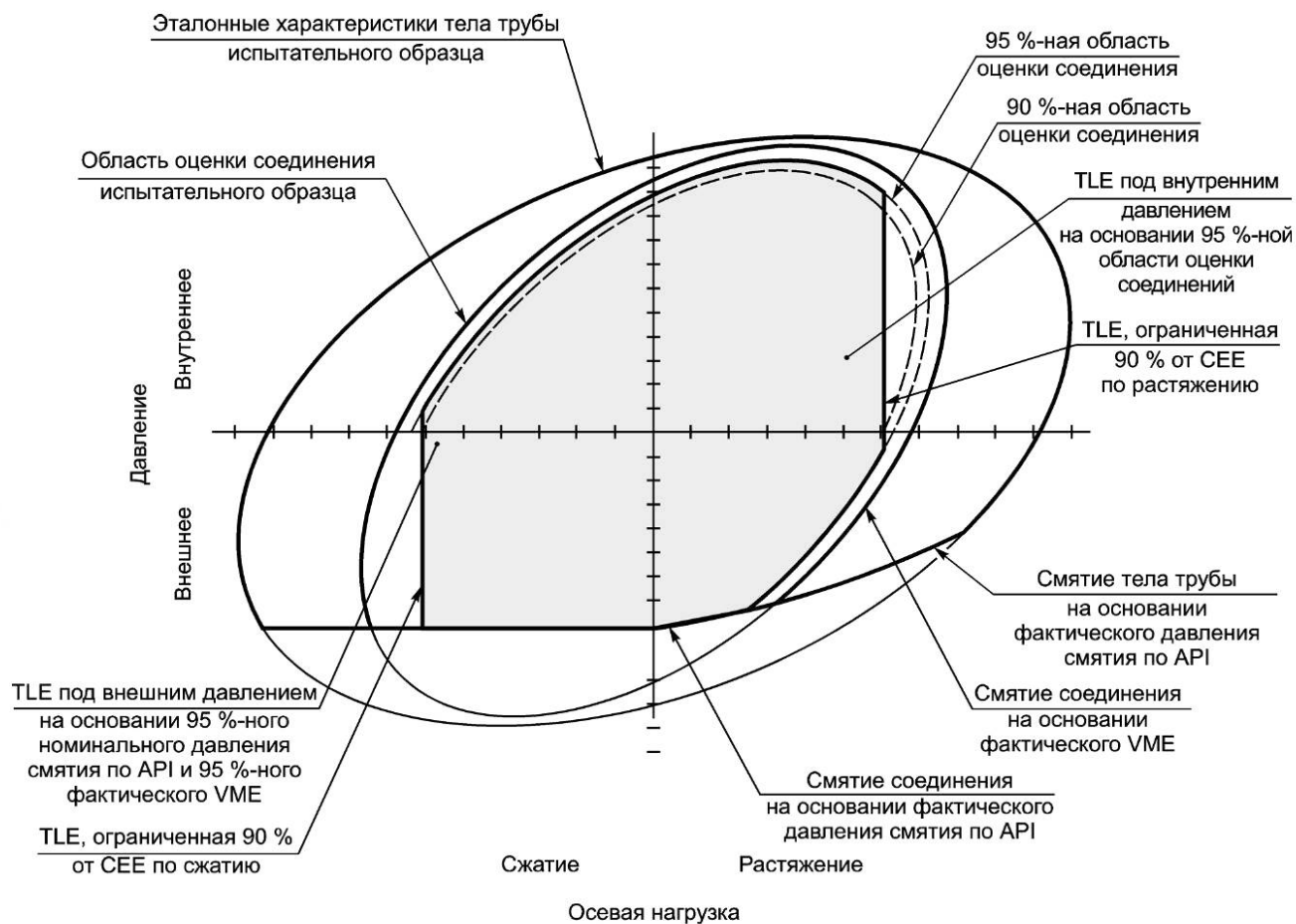
Рисунок 24 — Пример области испытательных нагрузок при несовпадении эталонных характеристик тела трубы и области оценки резьбового соединения и при TLE, составляющей 95 % от CEE для внутреннего давления и комбинации 95 % от фактического давления смятия по API и 95 % от фактического VME для наружного давления
