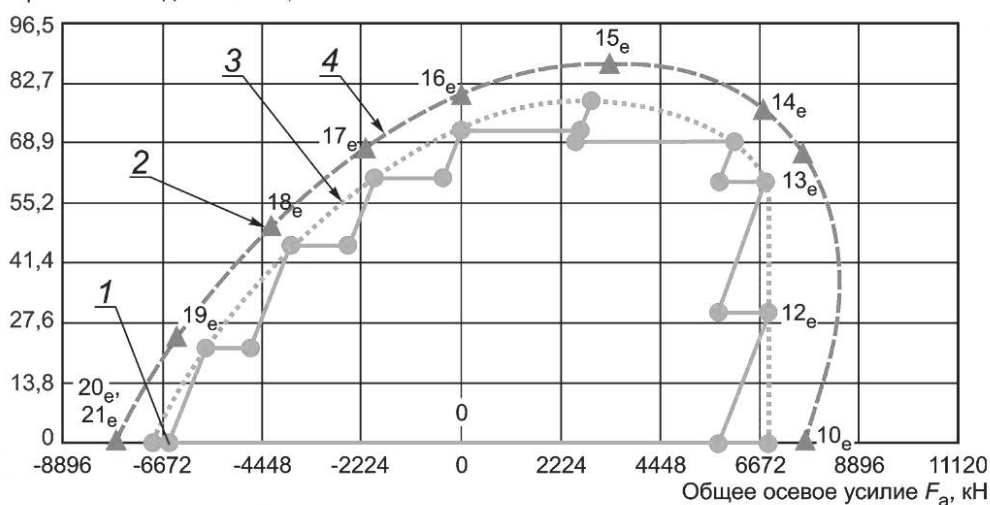
Рисунок D.26 — A e 90 % (QI, QII), TS-A этапы нагрузки 1—24
