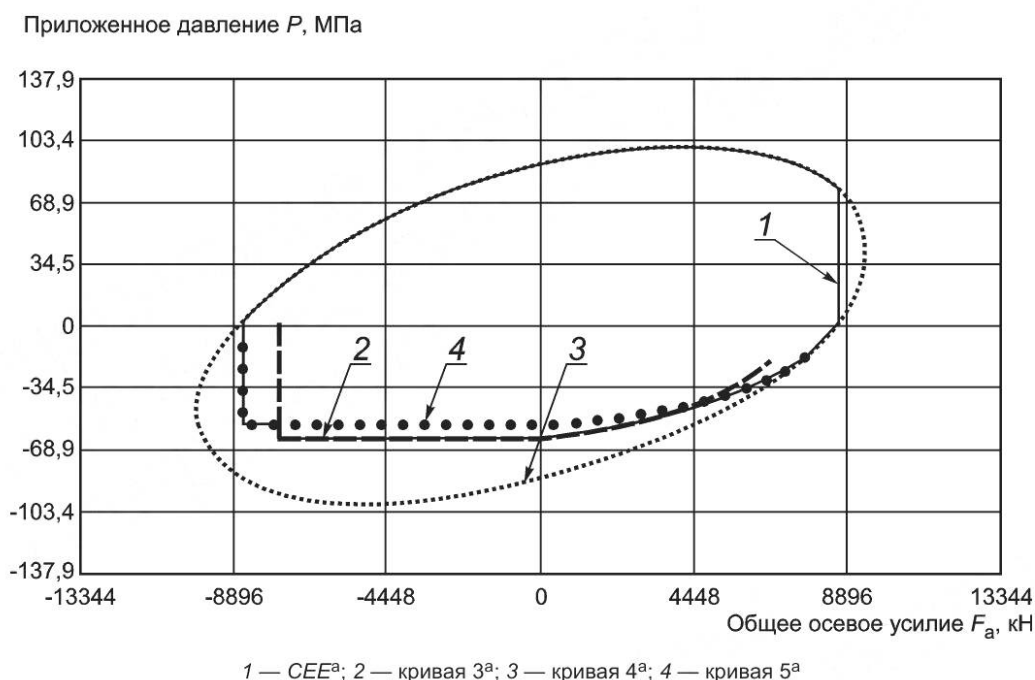
Рисунок D.14 — CEE^a испытательного образца при температуре окружающей среды
