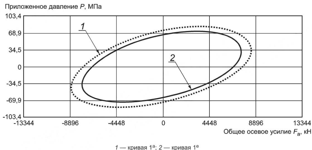
Рисунок D.9 — Кривые номинального VME испытательного образца тела трубы при температуре окружающей среды (1 a ) и при повышенной температуре (1 e )
