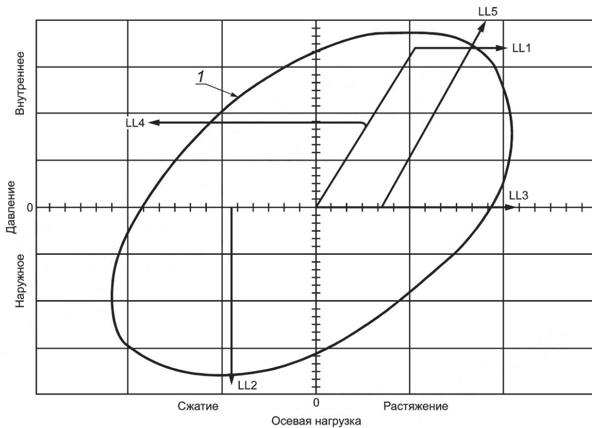
Рисунок 35 — Траектории приложения нагрузки при испытании при предельных нагрузках (пример 1)
