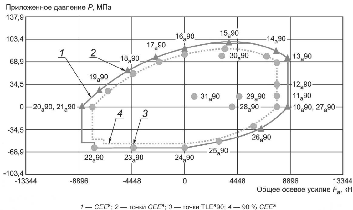
Рисунок D.18 — Точки CEE^a и точки нагрузки 90 % TLE^a при температуре окружающей среды
