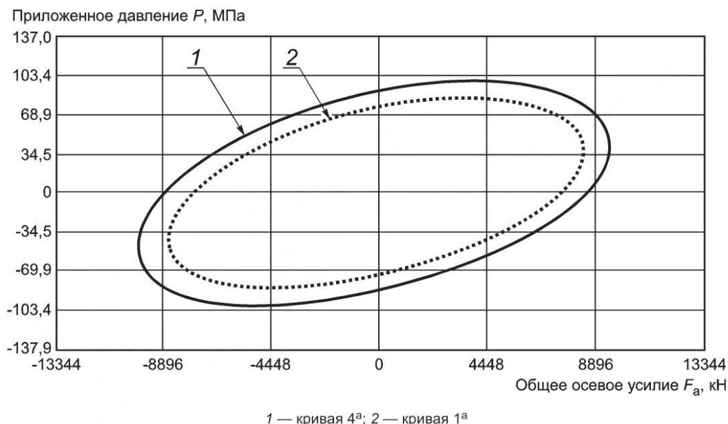
Рисунок D.7 — Кривые фактического (4 а ) и номинального (1 а ) VME испытательного образца тела трубы при температуре окружающей среды
