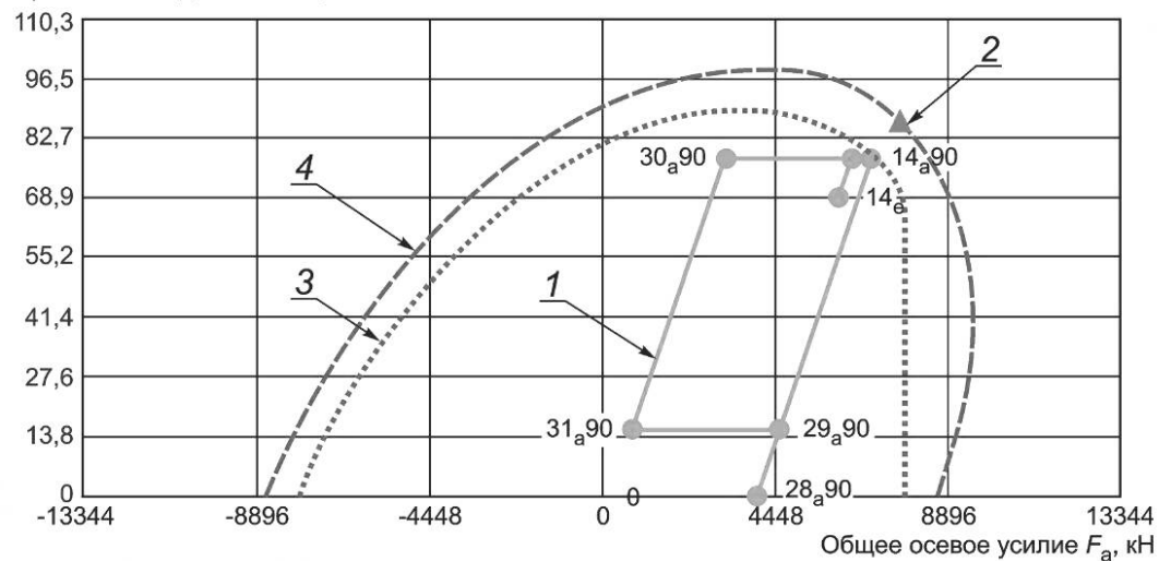
Рисунок D.25 — Пять механических циклов, TS-C этапы нагружки 45—69
