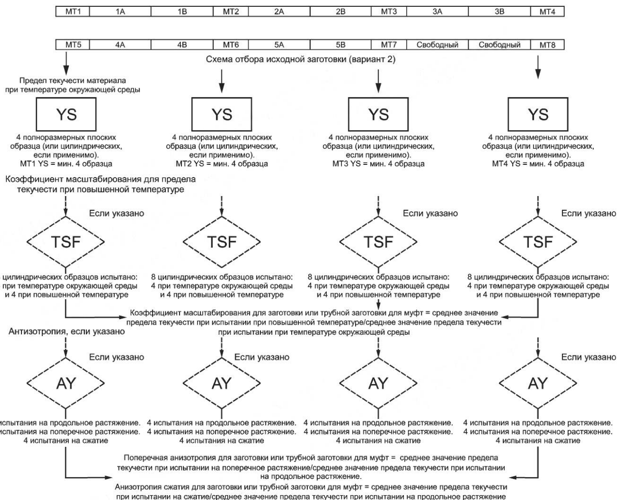
Рисунок D.2 — Схематическое представление требований к проведению механических испытаний
