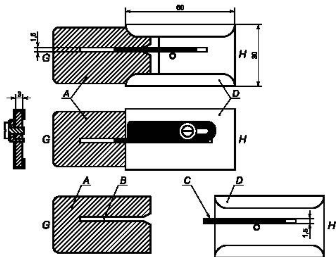
А — стальная пластина; В — прорез; С — стальной язычок; D — направляющие
