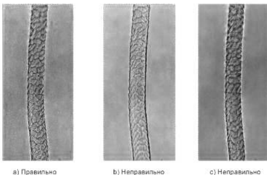
Рисунок 5 — Правильно и неправильно сфокусированные волокна
