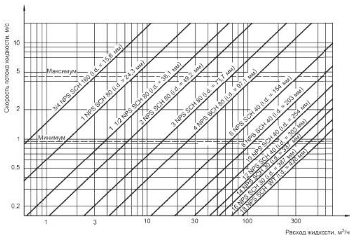
Рисунок 2 — Скорость в жидкостных трубопроводах
