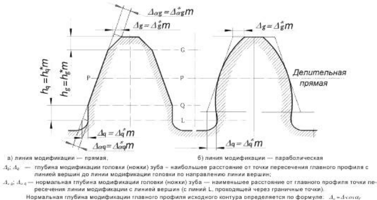
Рисунок ДА.2 — Общие схемы модификации исходного контура
