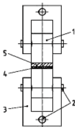
1 – испытательная сборка; 2 – штифты; 3 – хомут; 4 – адгезивный связующий материал; 5 – испытуемое покрытие
