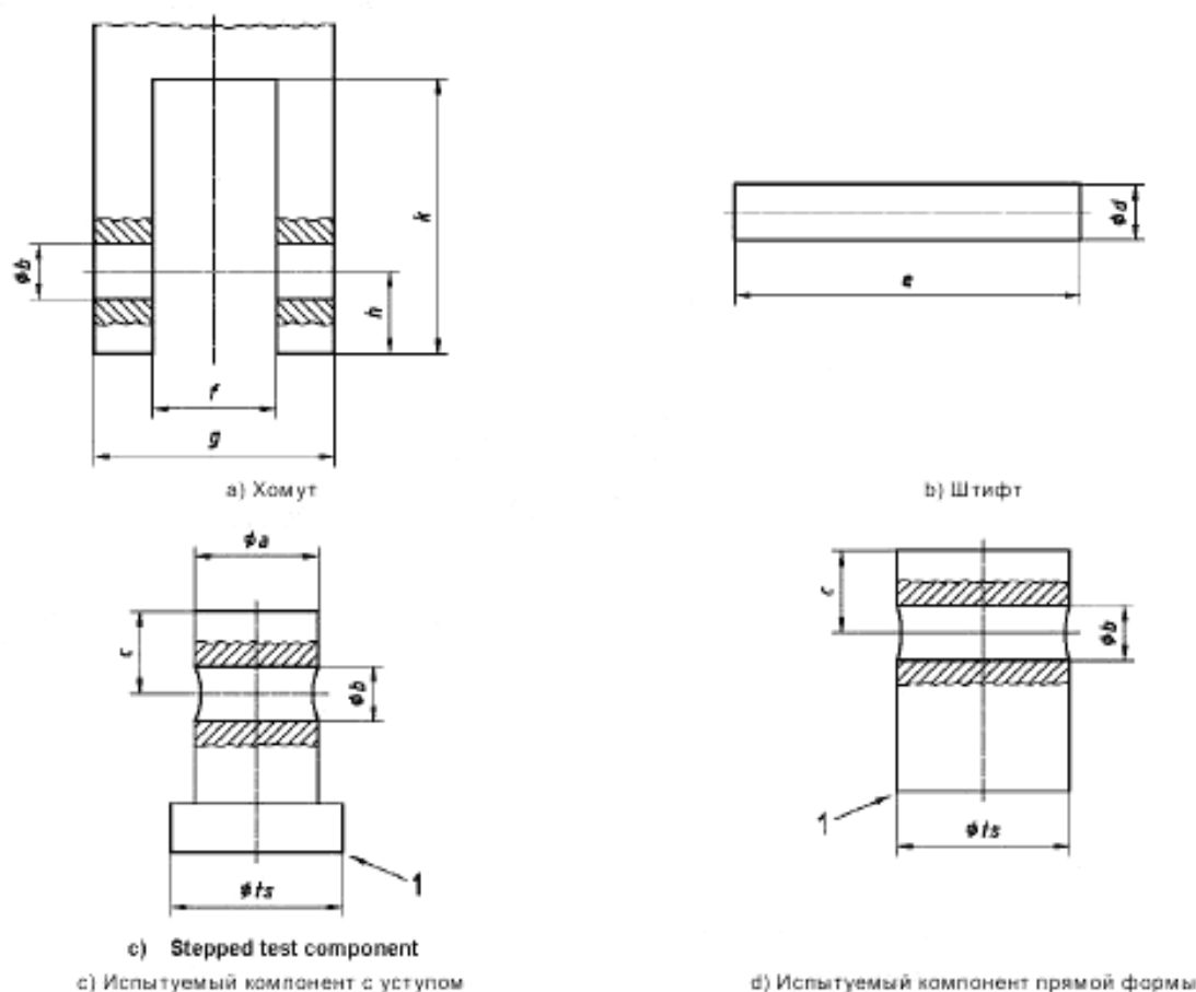
Рисунок 2 – Размеры нагрузочного блока и испытываемых компонентов
