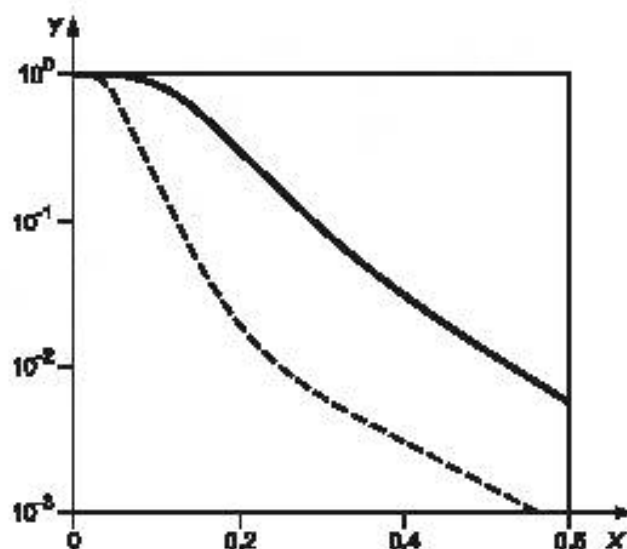
X — максимальная скорость, м/с; Y — вероятность превышения за год, P_0 ; — город А; --- город В
