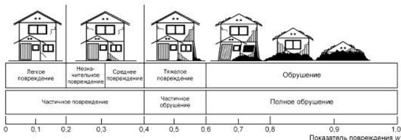
Рисунок Н.1 — Степень и показатель повреждения
