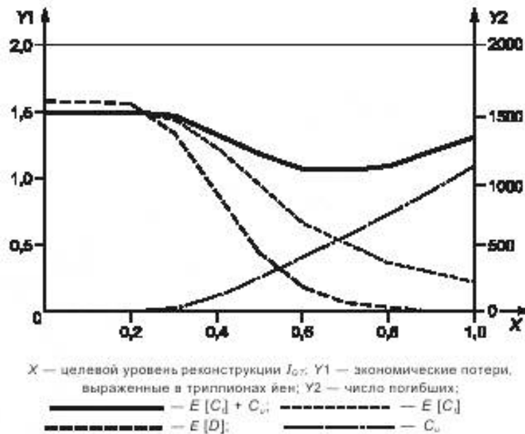
Рисунок H.2 — Целевой уровень и ожидаемые потери
